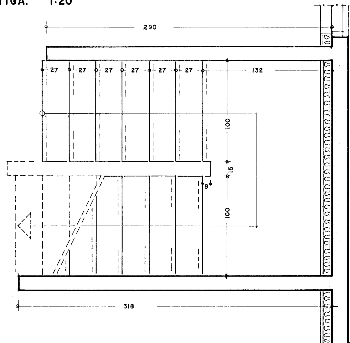
GRUNNMYND STIGA 1:20
