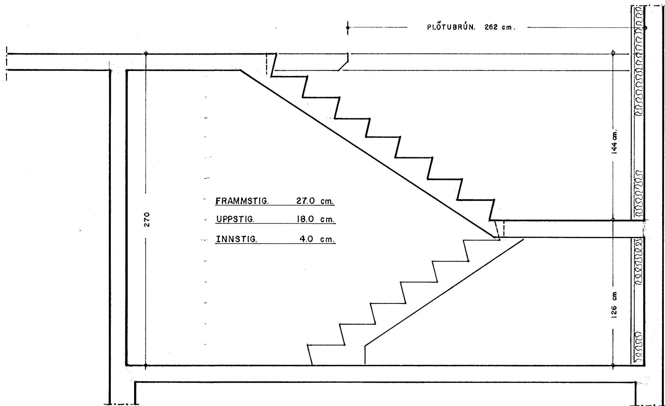
SNEIÐING Í STIGA. 1:20
