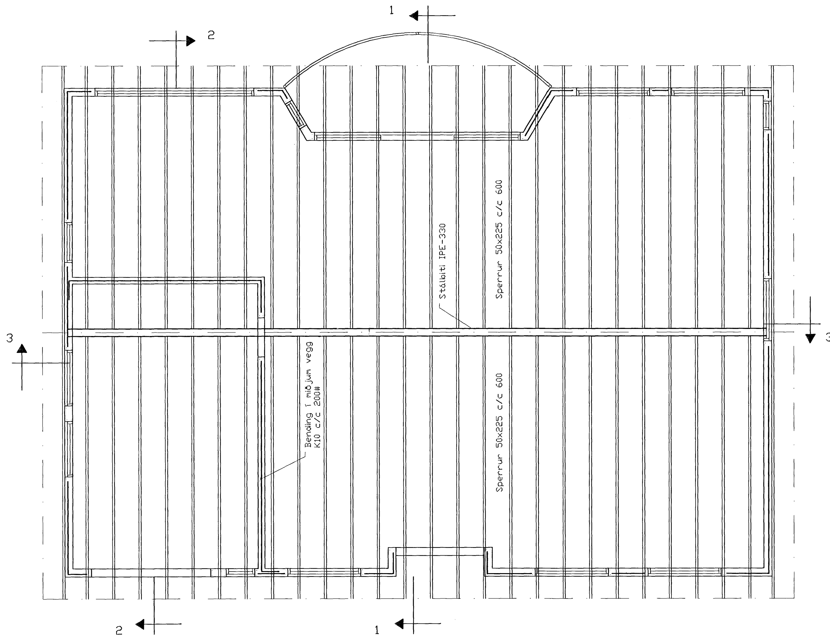
Grunnmynd, 1:50
