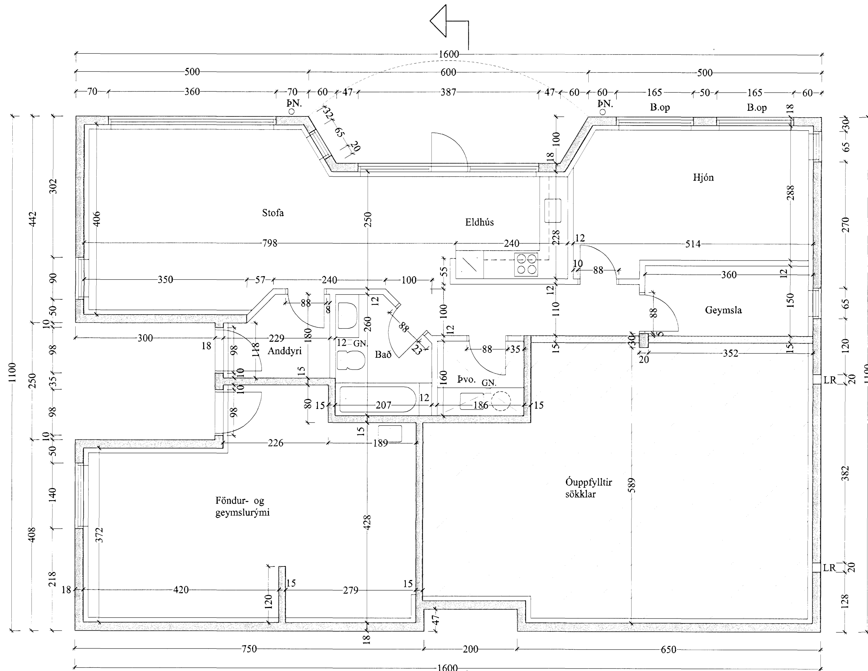
GRUNNMYND 1. HÆÐ M 1:50
