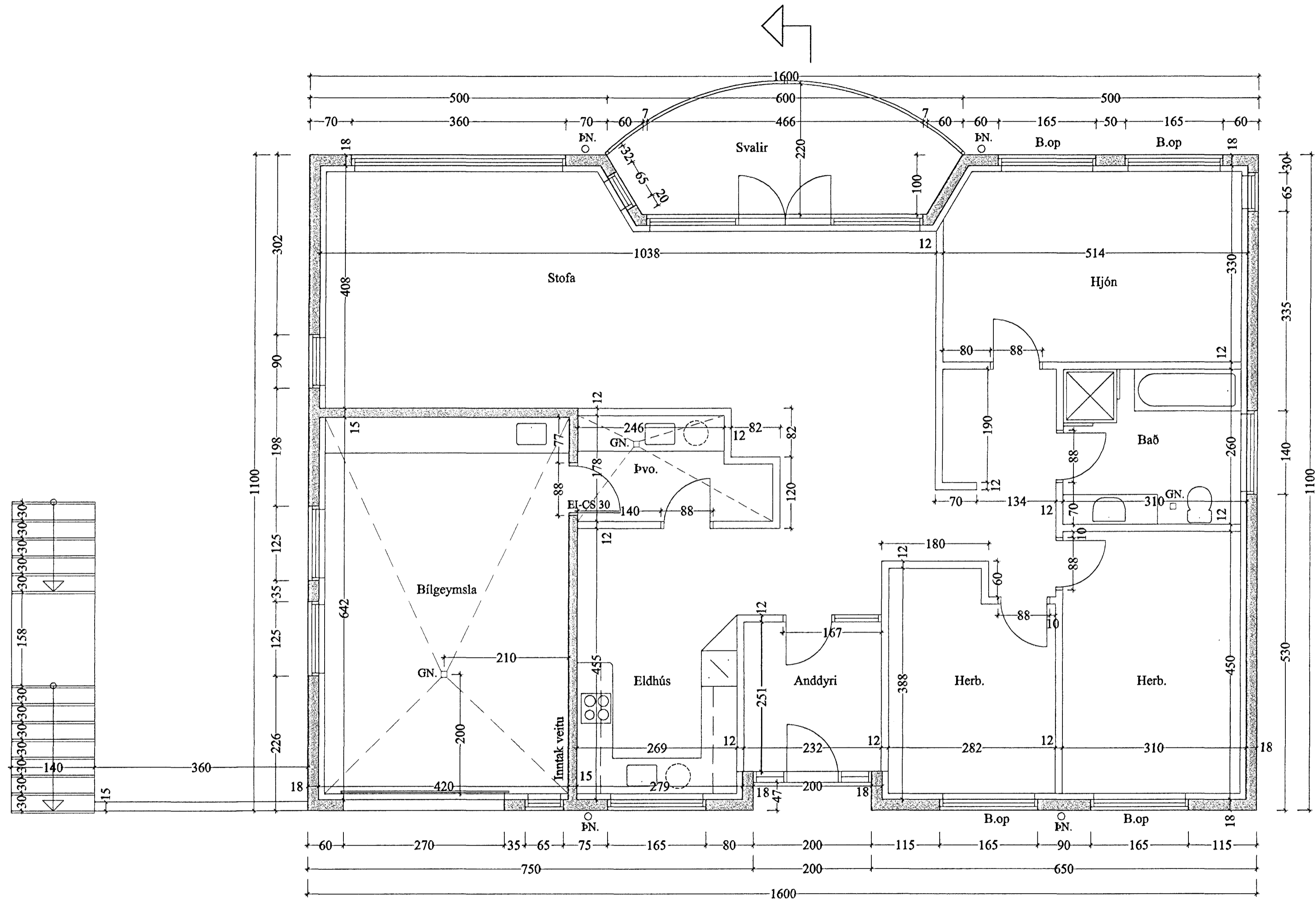
GRUNNMYND 2. HÆÐ M 1:50
