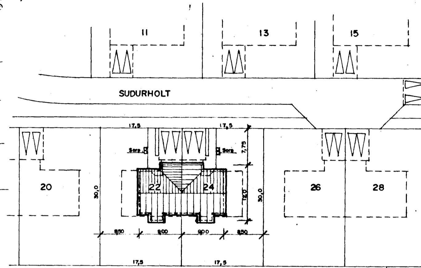
AFSTÖÐUMYND 1:500
