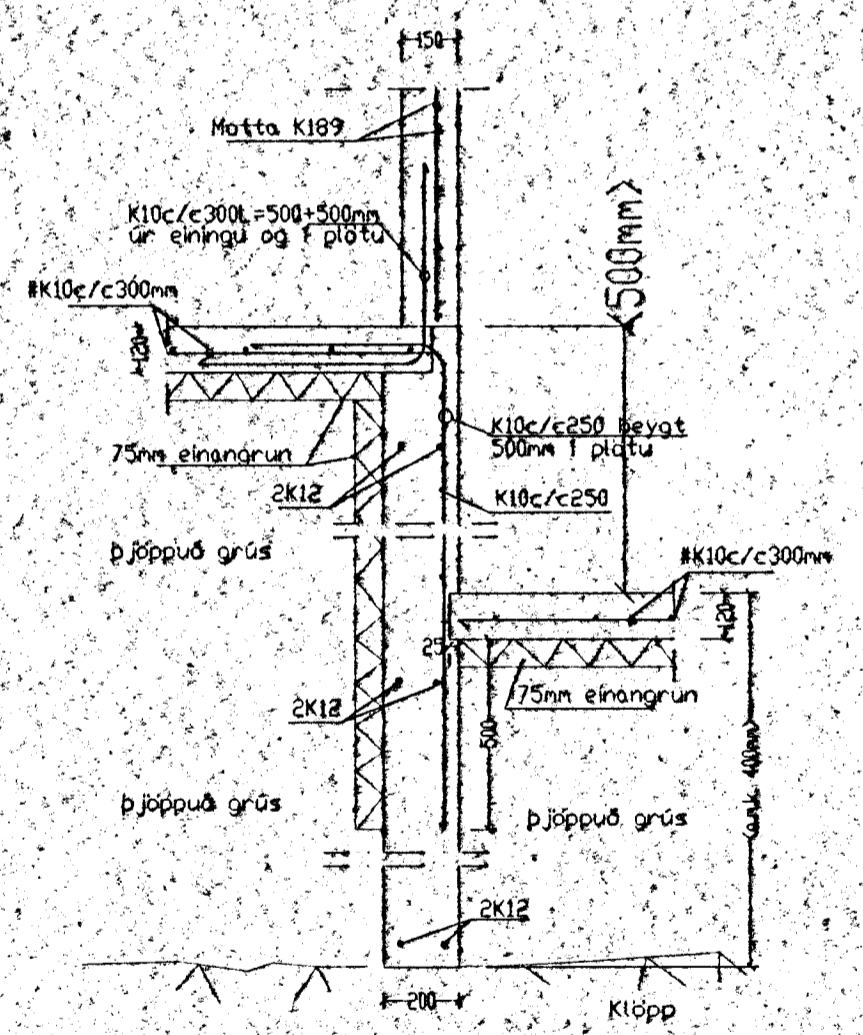
Snið A5 1:20
