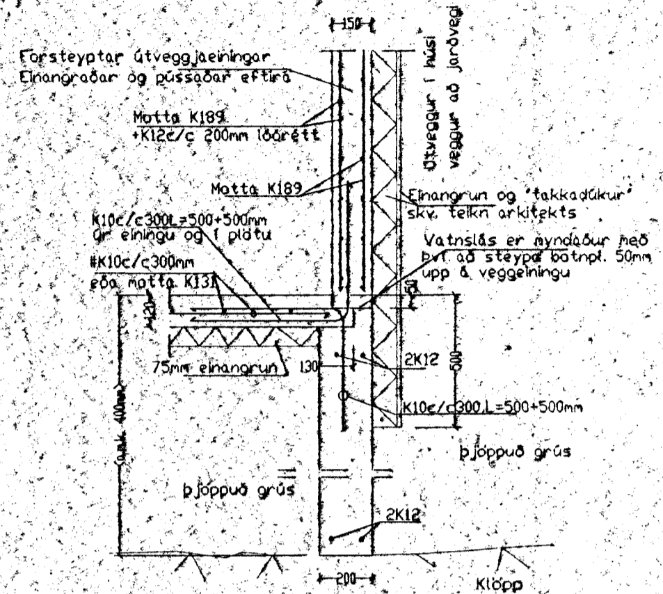
Snið A1 1:20
