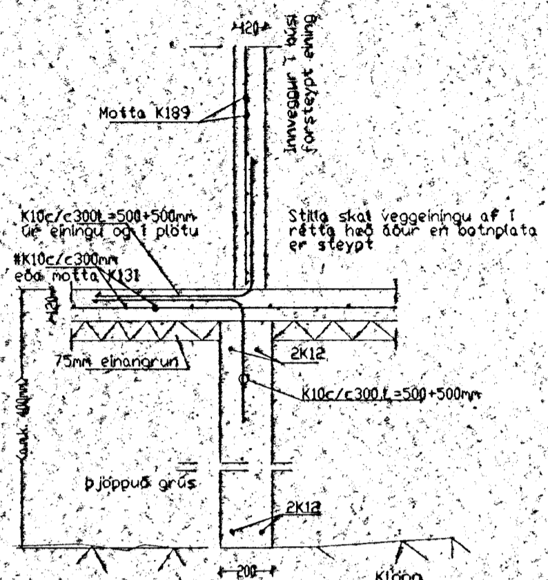
Snið A2 1:20
