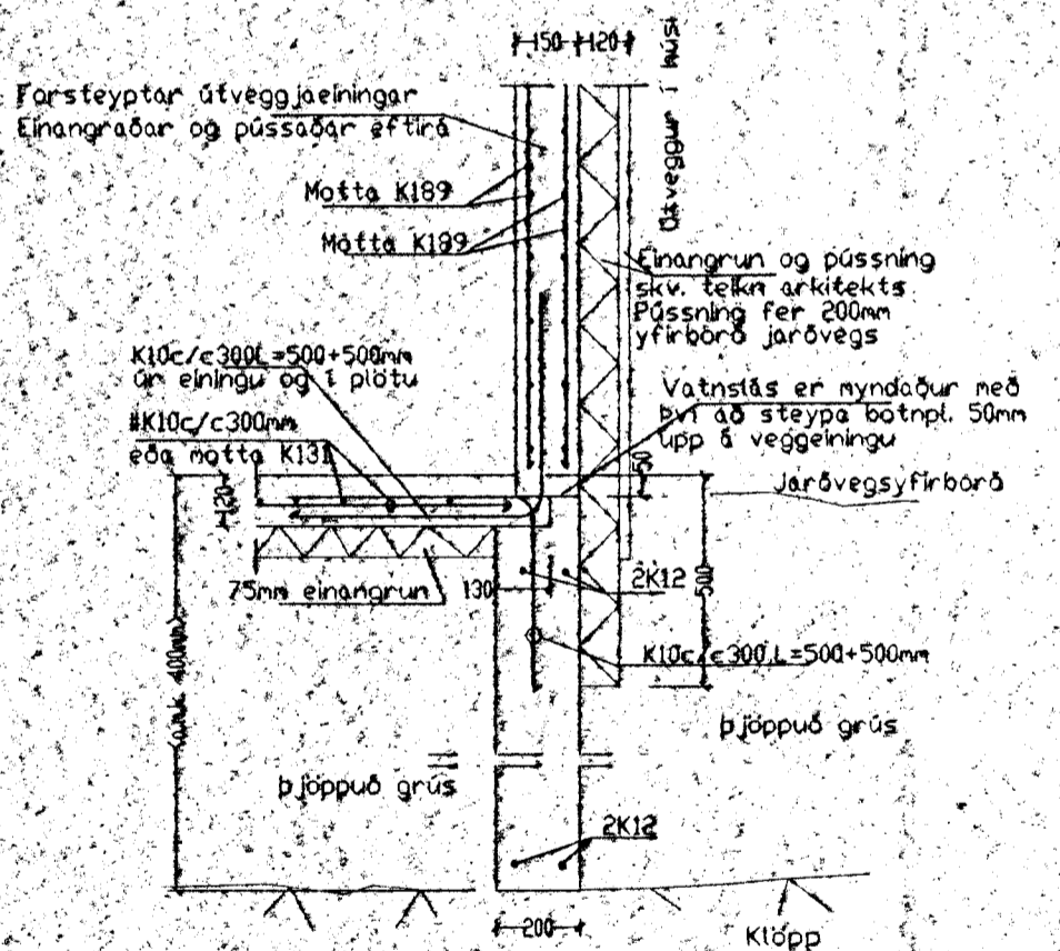
Snið A4 1:20
