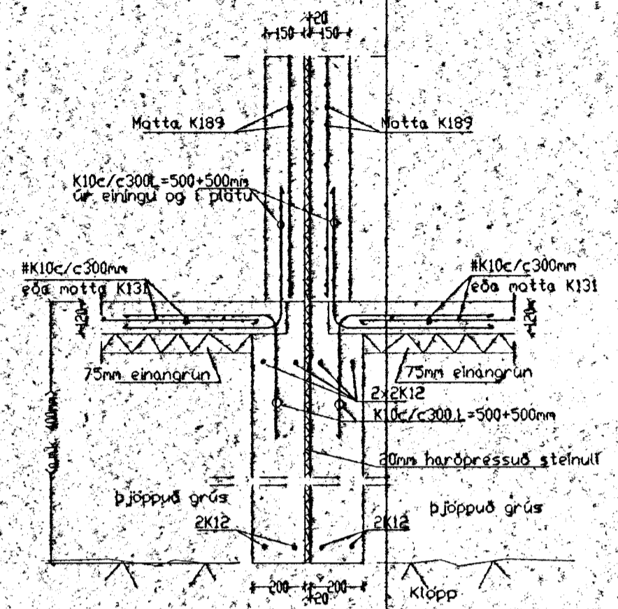
Snið A3 1:20
