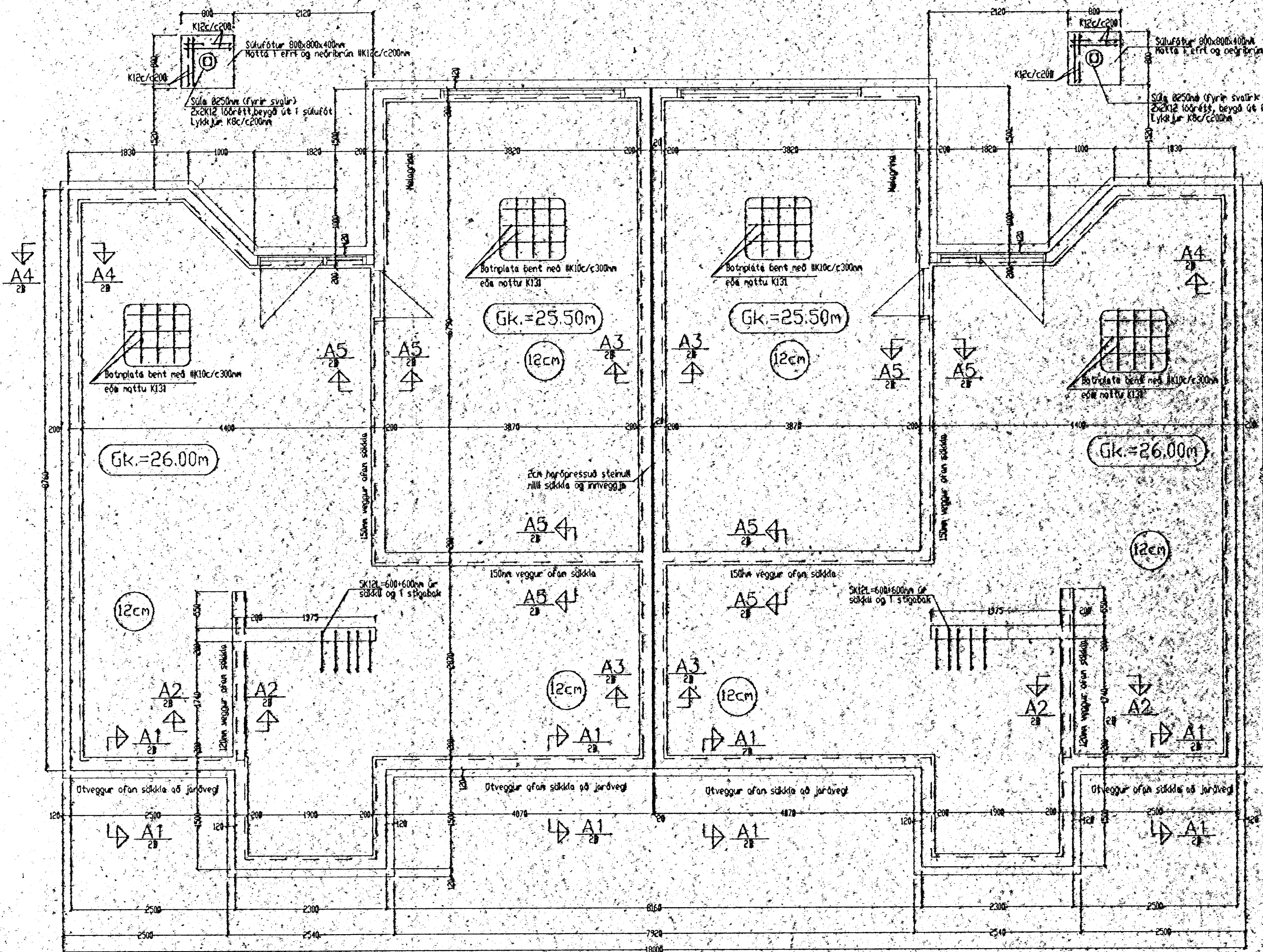
Grunnmynd sökklá 1:50
