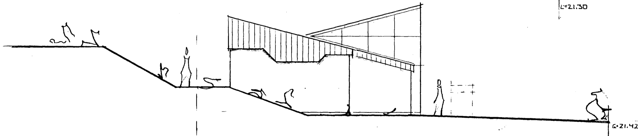
ÚTLIT NORÐUR 1:100
