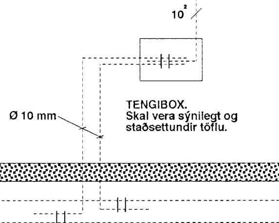
SNID Í TÖFLUVEGG
