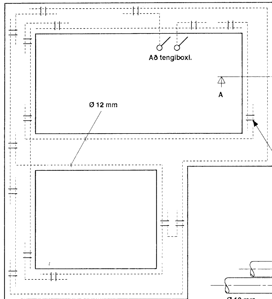
Almenn grunnmynd sökkulvegja.
