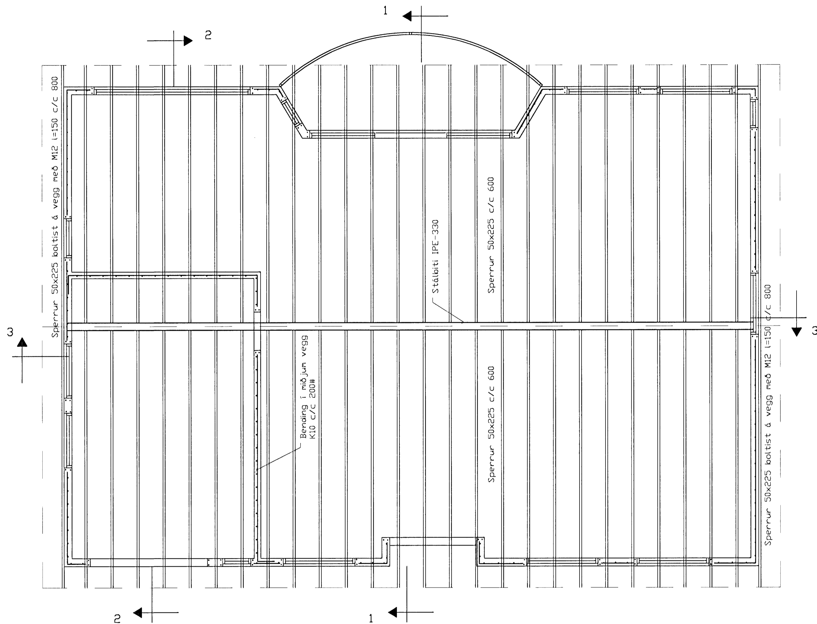
Grunnmynd, 1:50
