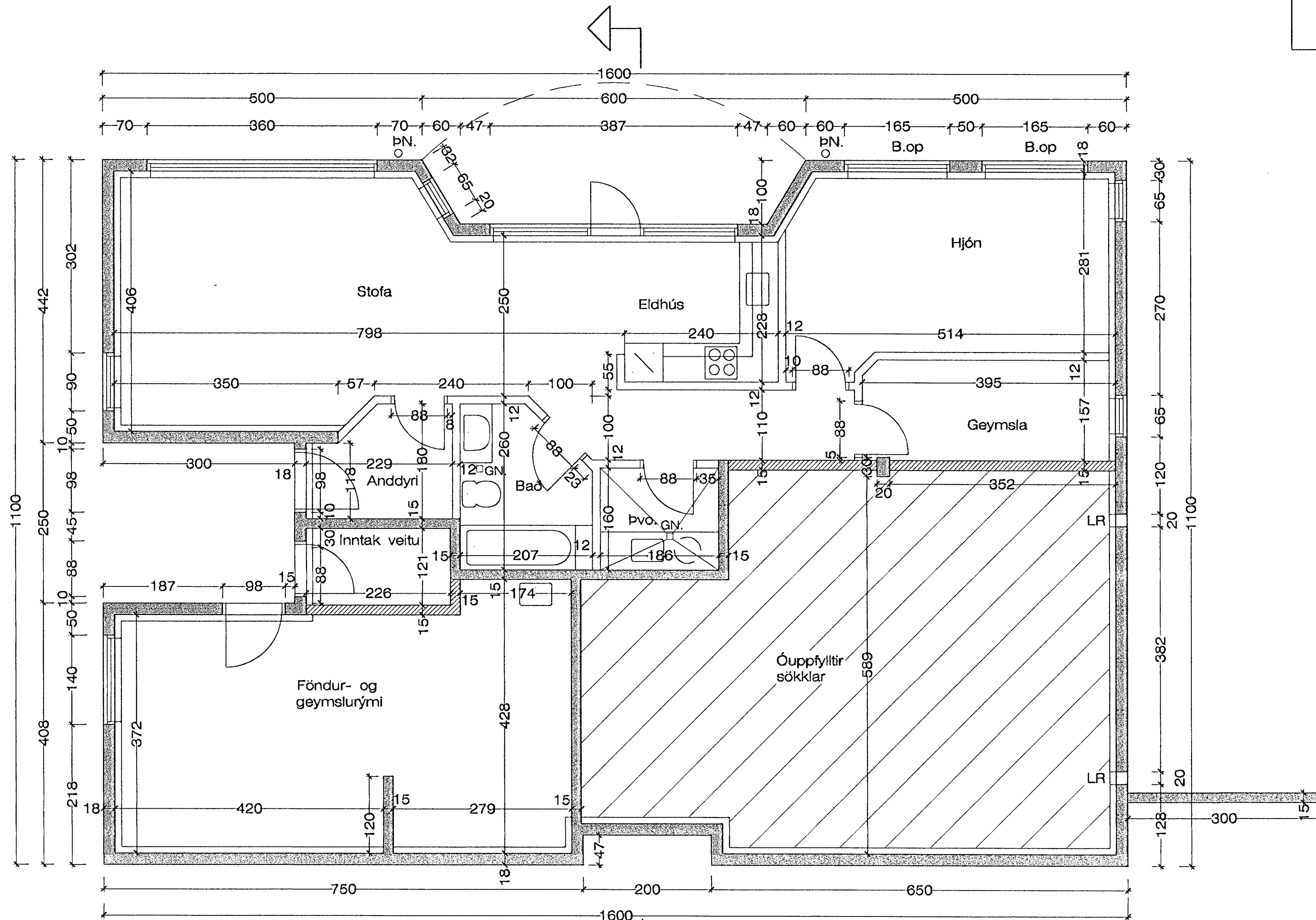
GRUNNMYND KJALLARI M 1 : 50
