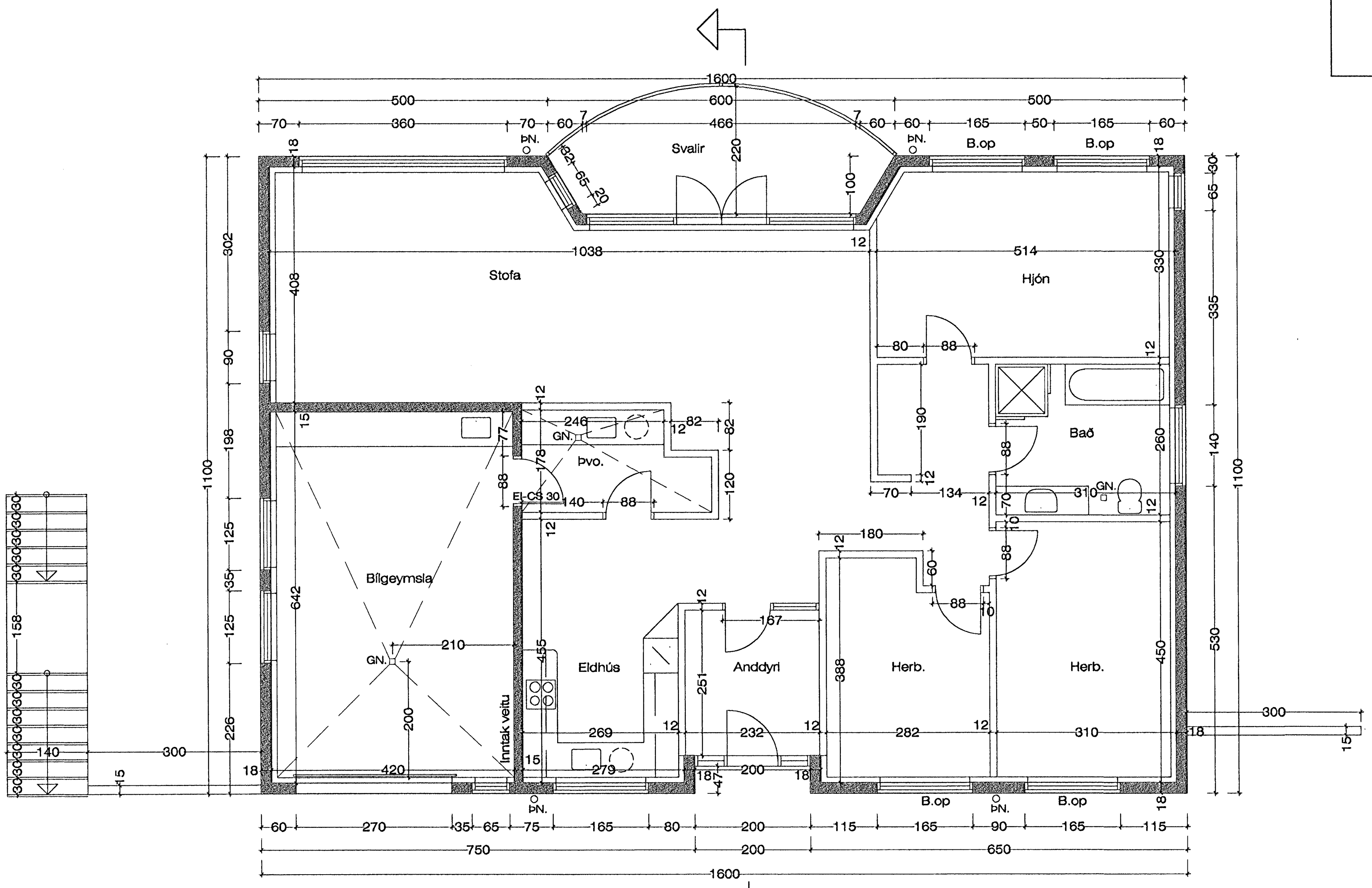
GRUNNMYND 1. HÆÐ M 1:50
