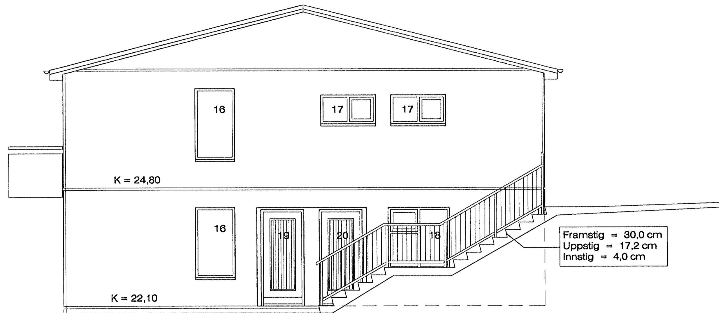
ÚTLIT SUÐAUSTUR M 1 : 50
