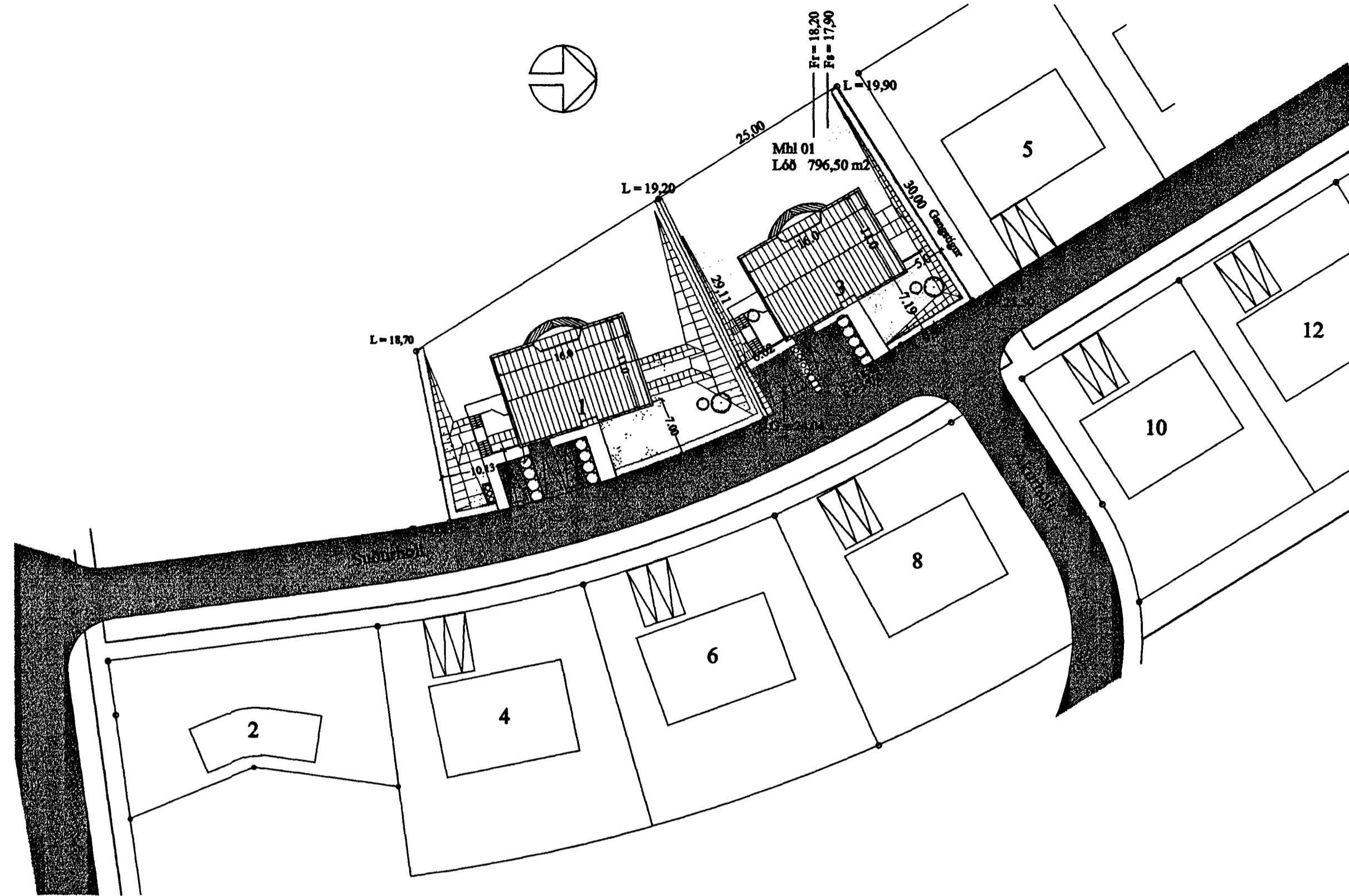
AFSTÖÐUMYND M 1 : 500
