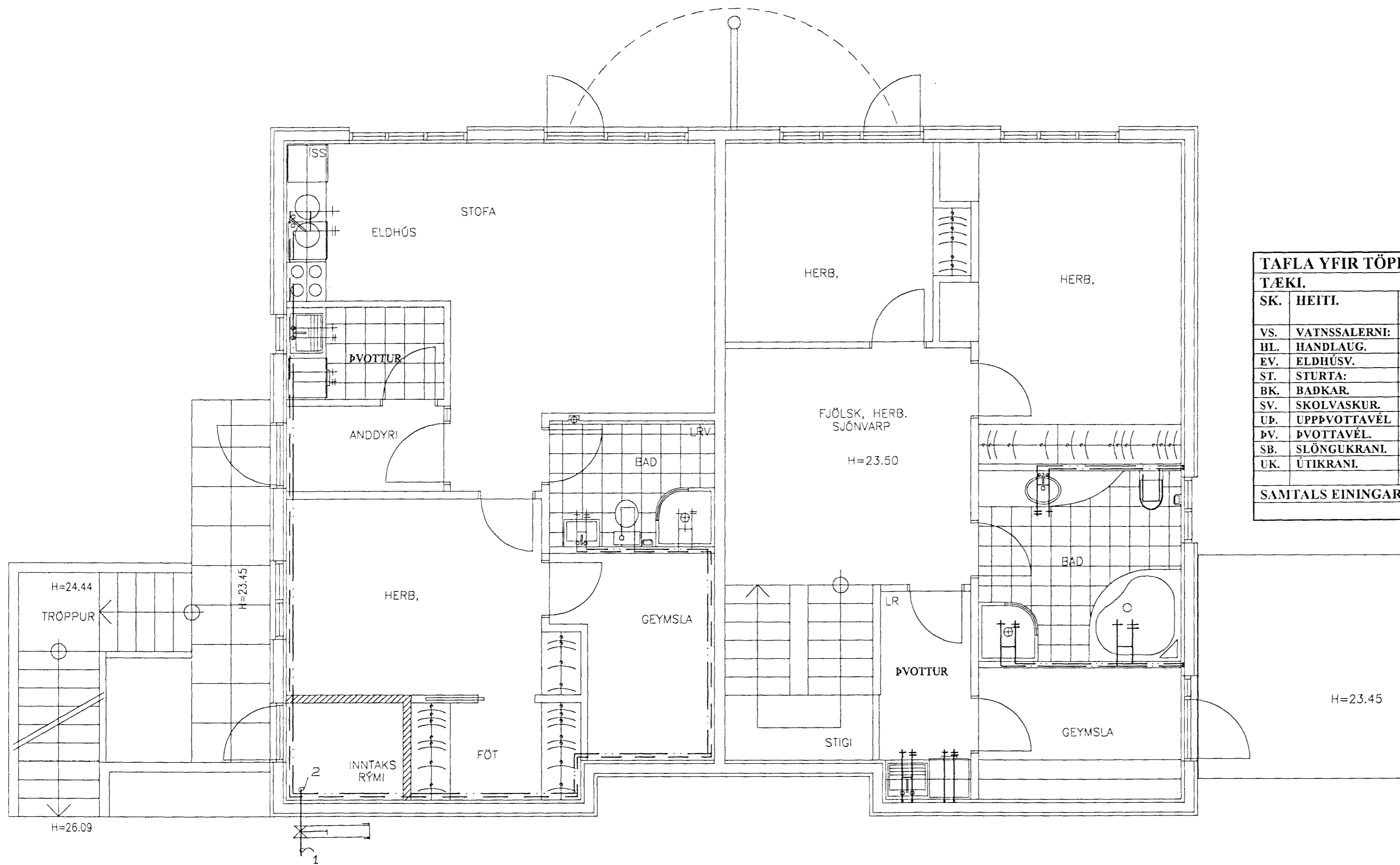
GRUNNMYND NEDRI HÆD – MKV 1:50
