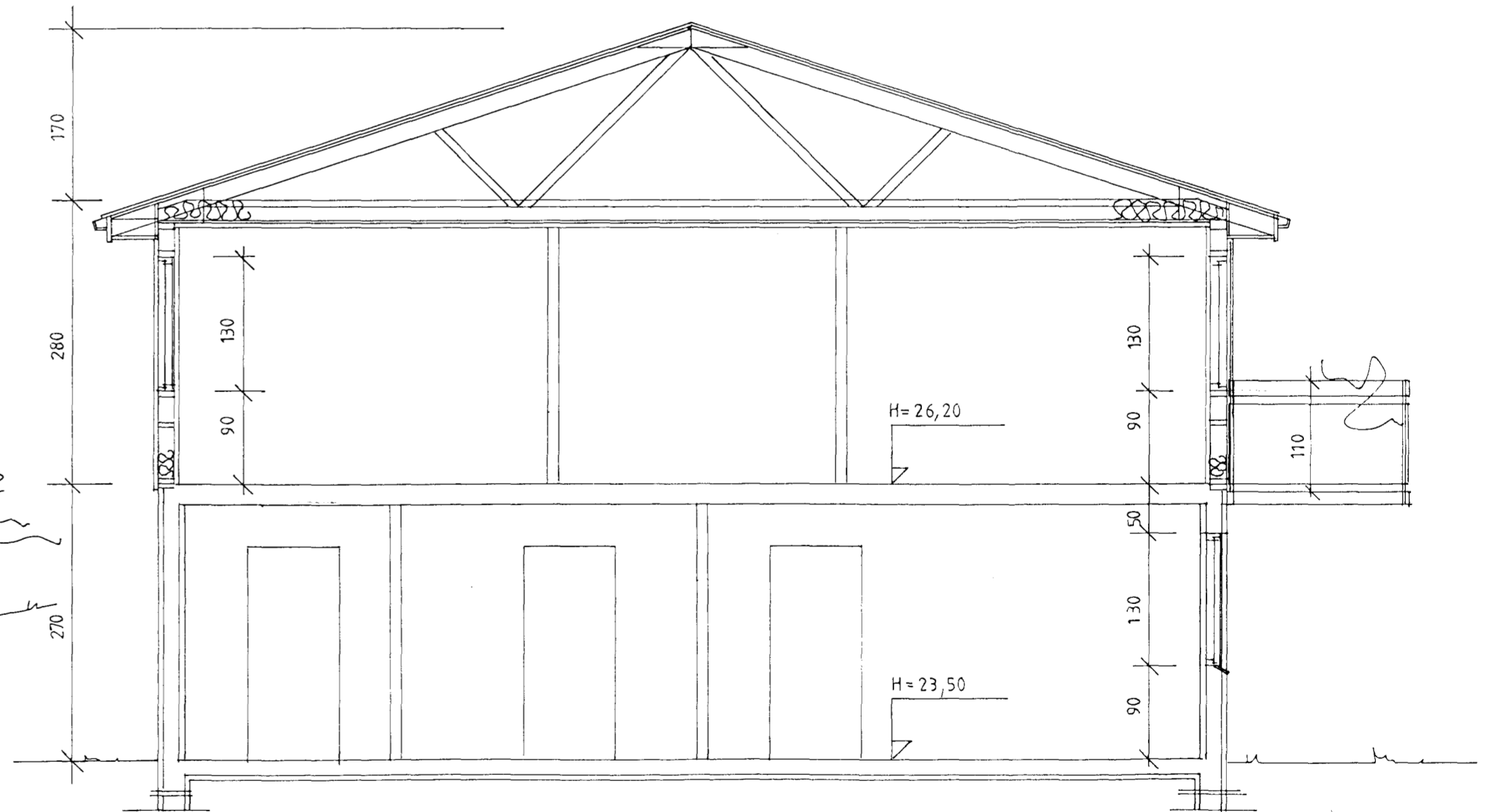
SNID A-A
