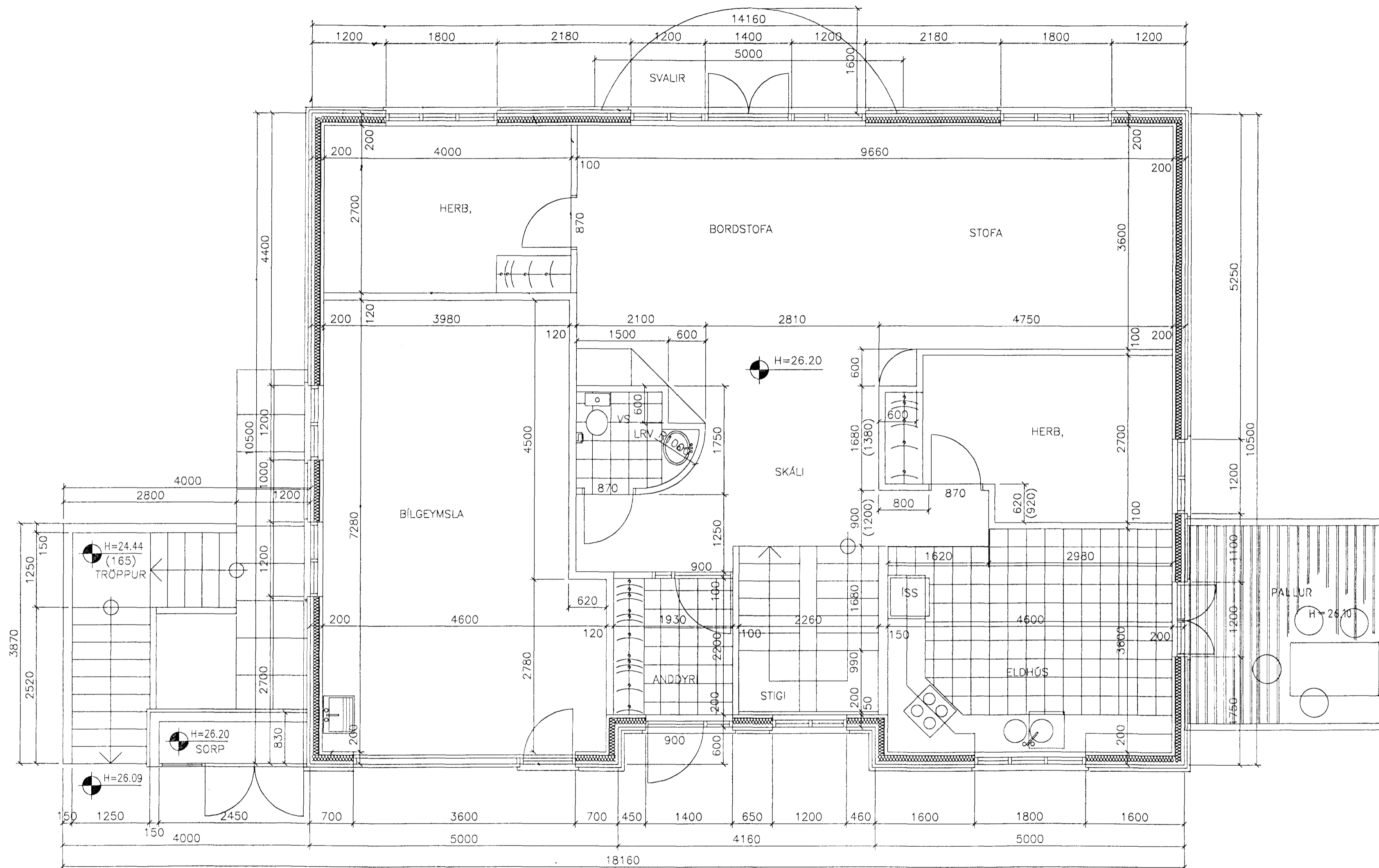
GRUNNMYND EFRI HÆÐ - MKV 1:50
