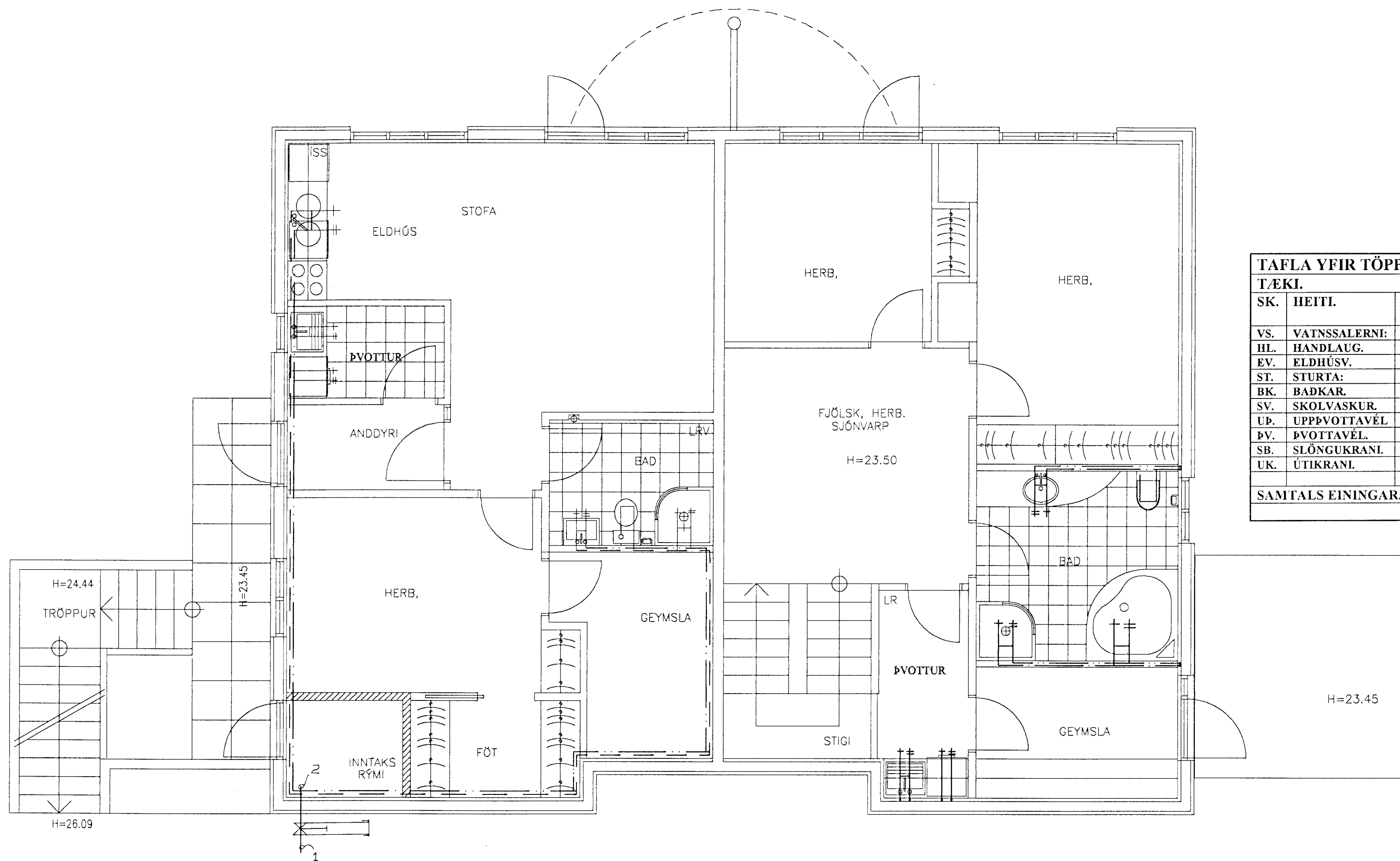
GRUNNMYND NEDRI HÆÐ – MKV 1:50
