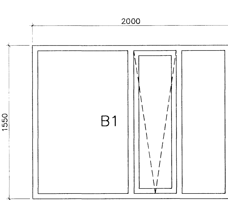
1 STK. GLUGGI-OPNANLEGUR
