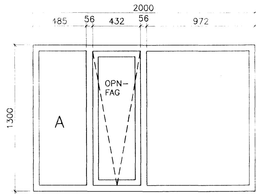
2 STK. GLUGGAR-OPNANLEGIR
