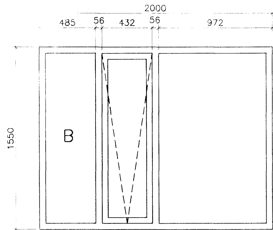
1 STK. GLUGGI-OPNANLEGUR
