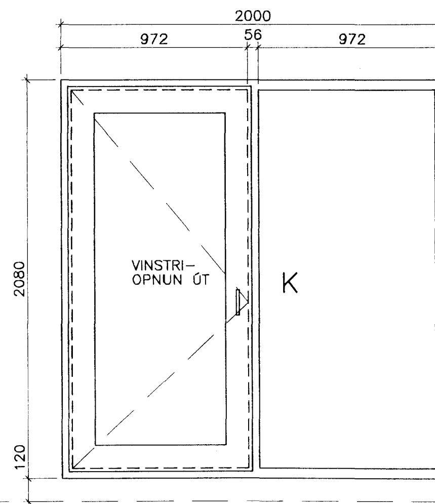
2 STK. GLUGGAR/SVALAHURDIR
