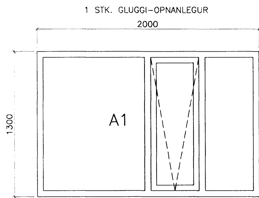
1 STK. GLUGGI-OPNANLEGUR
