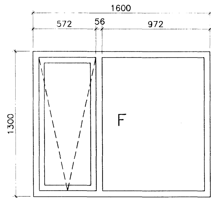
1 STK. GLUGGI-OPNANLEGUR
