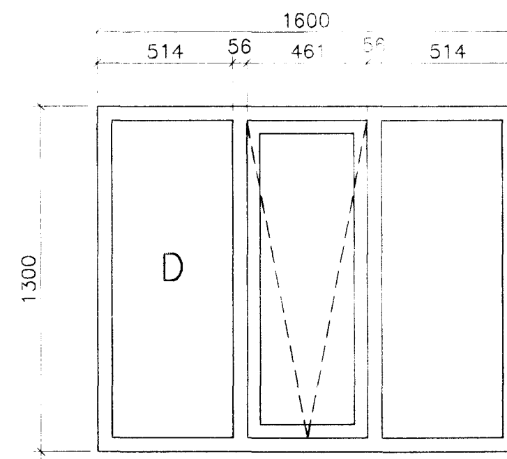
7 STK. GLUGGAR-OPNANLEGIR
