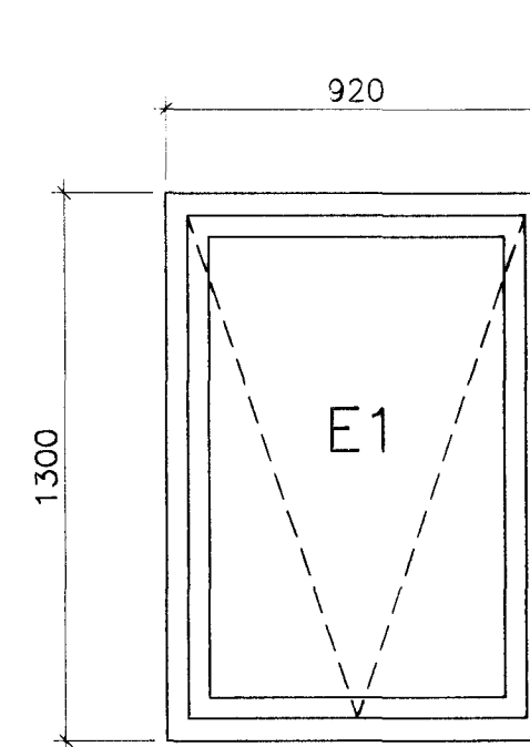
1 STK. GLUGGI-OPNANLEGUR
