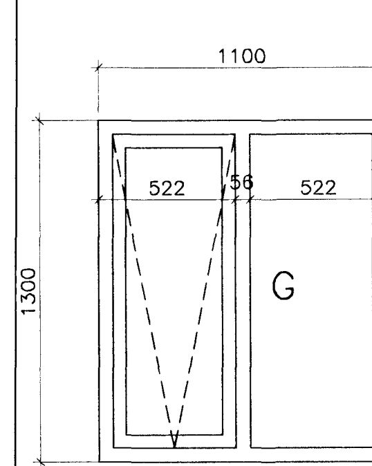
1 STK. GLUGGI-OPNANLEGUR
