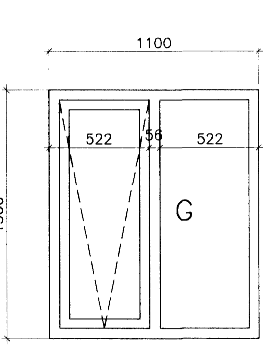
1 STK. GLUGGI-OPNANLEGUR
