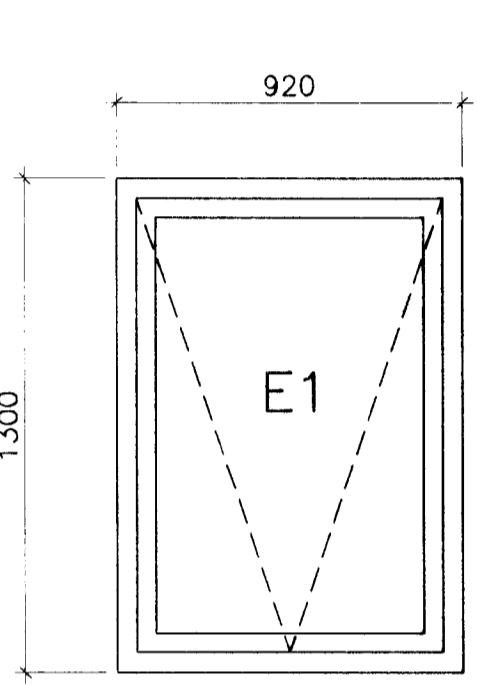
1 STK. GLUGGI-OPNANLEGUR
