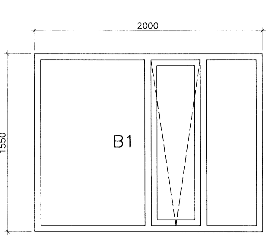
1 STK. GLUGGI-OPNANLEGUR
