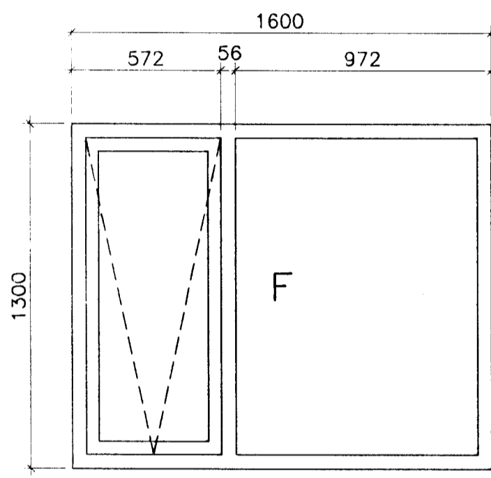
1 STK. GLUGGI-OPNANLEGUR
