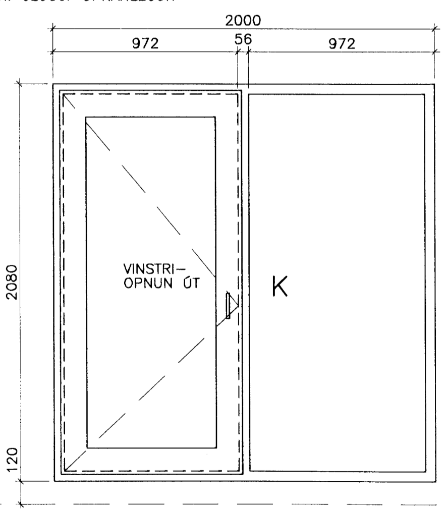
2 STK. GLUGGAR/SVALAHURDIR
