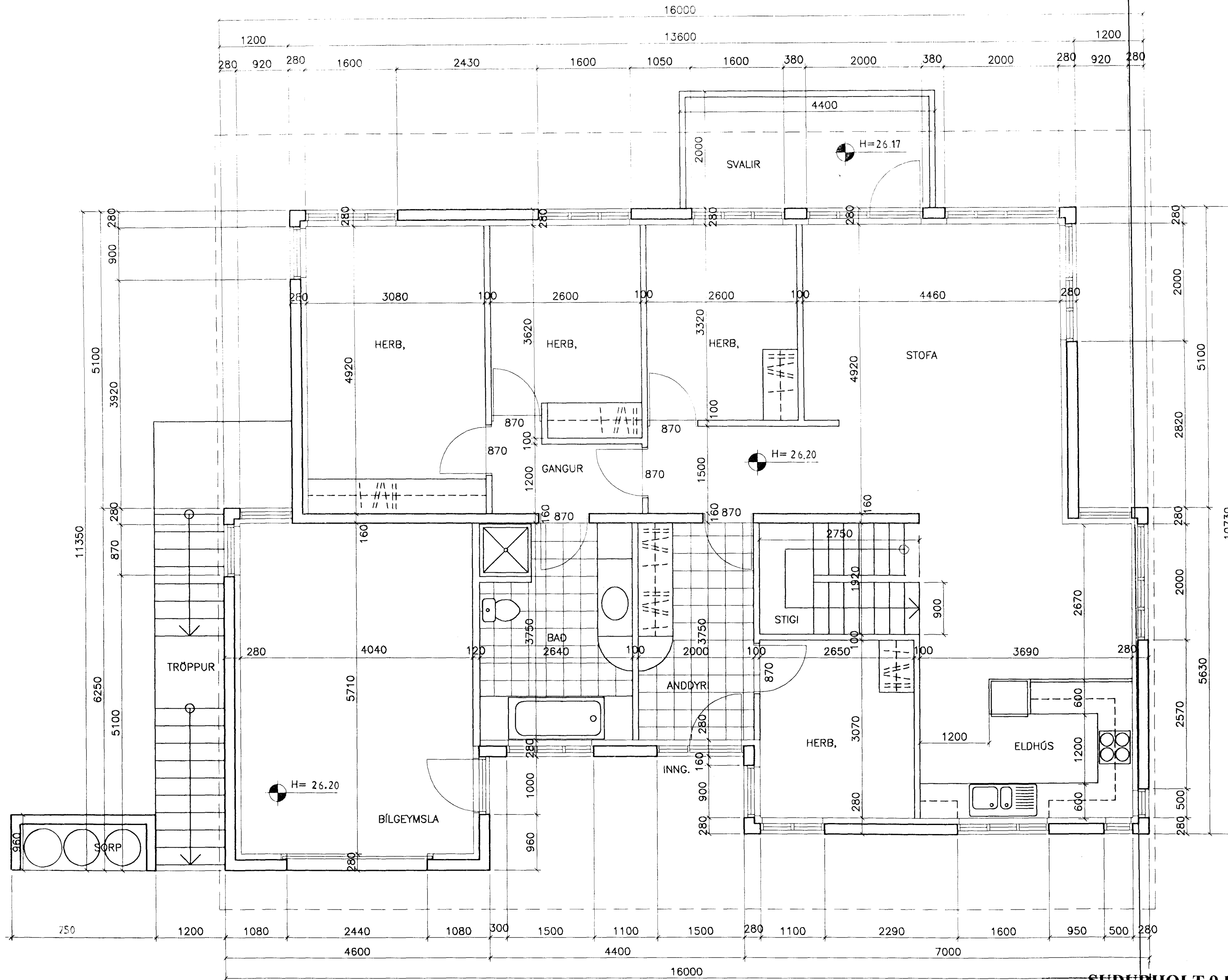
GRUNNMYND EFRI HÆÐ — MKV 1:50
