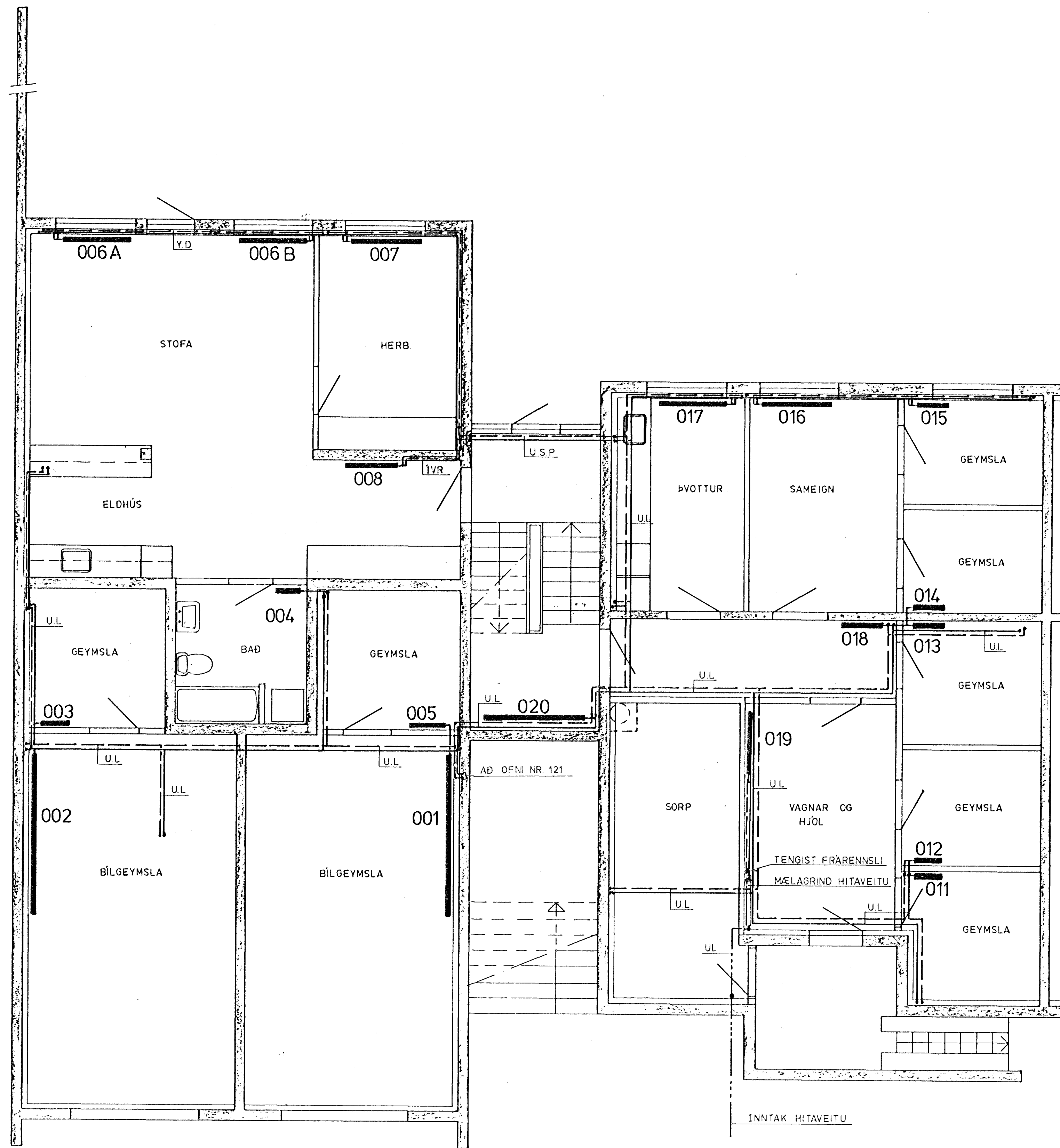
GRUNNMYND JARÐHÆÐAR 1 : 50
