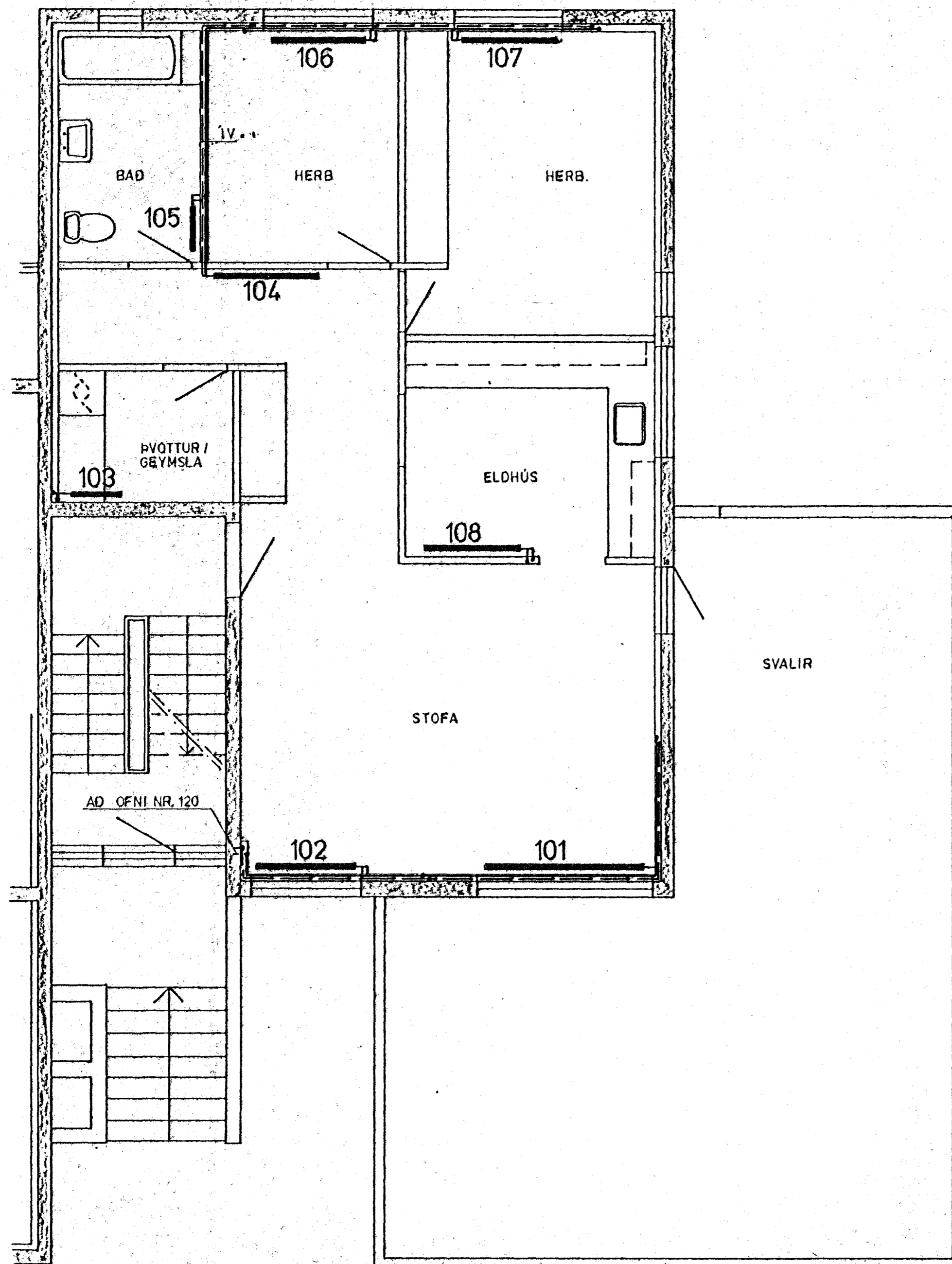
GRUNNMYND 1. HÆÐAR 1:50
