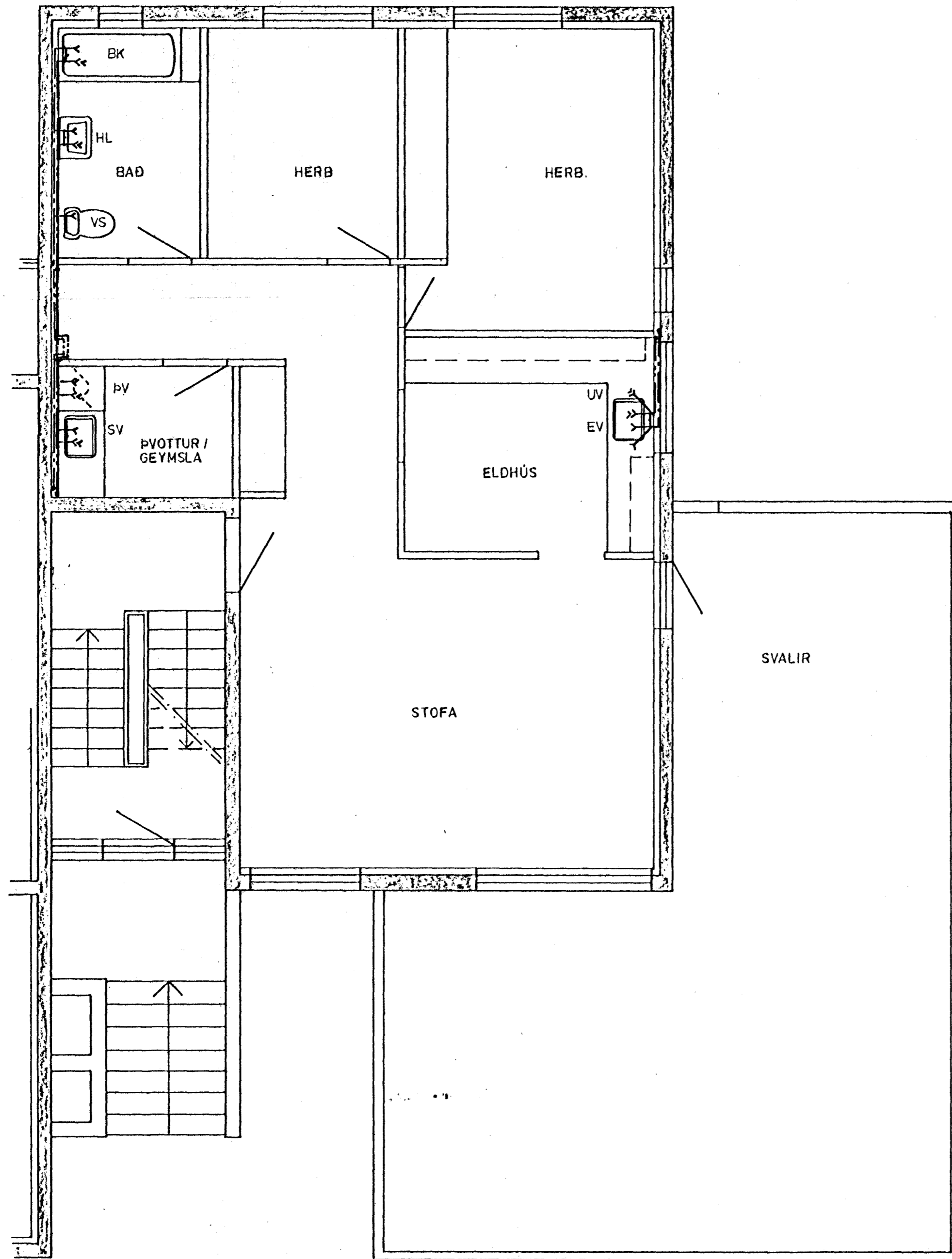
GRUNNMYND 1. HÆÐAR 1:50
