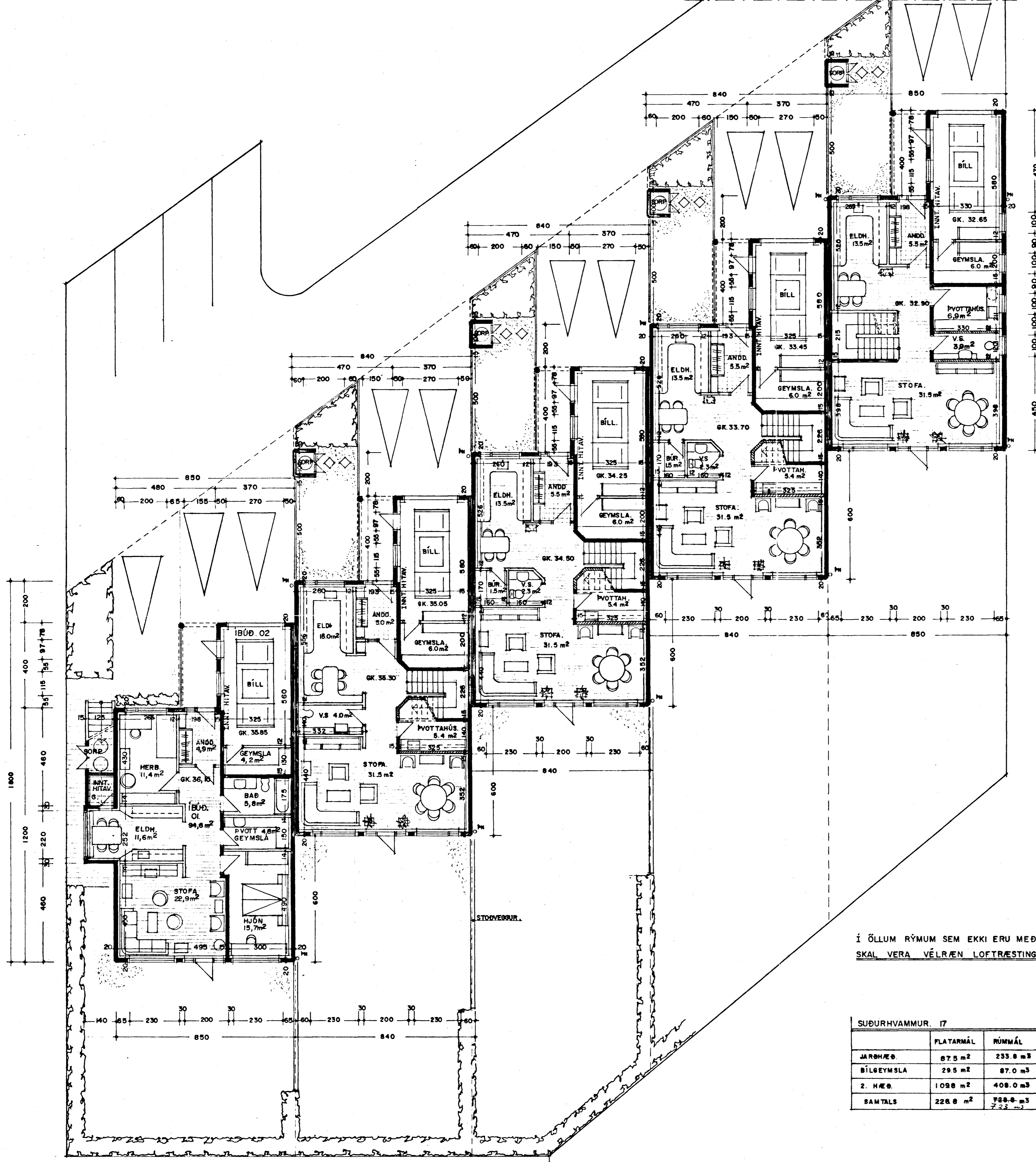
GRUNNMYND JARÐHÆÐAR. 1:100
