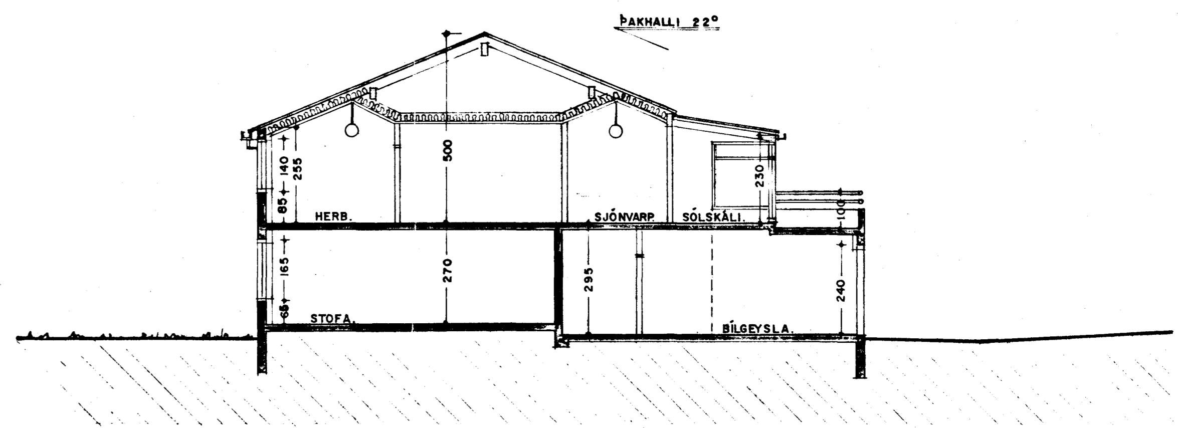
SNEIÐING B - B
