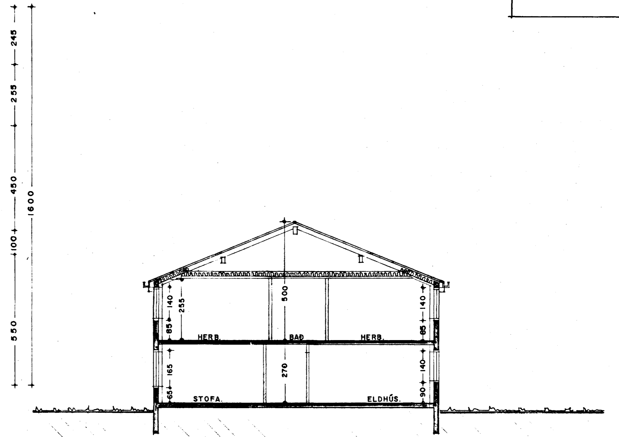
SNEIÐING A - A
