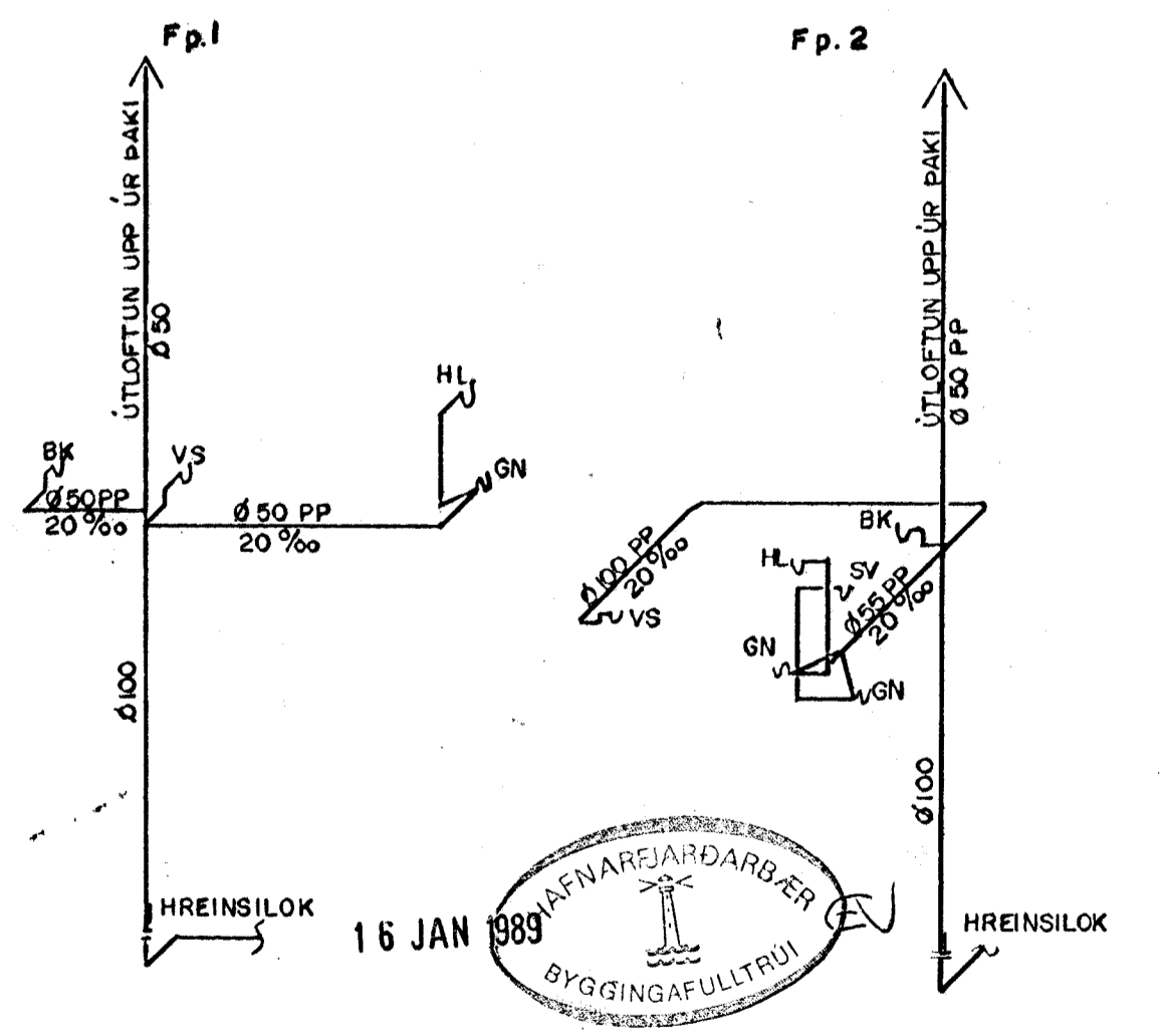
RÚMMYND LAGNA INNI Í HÚSI 1:50
