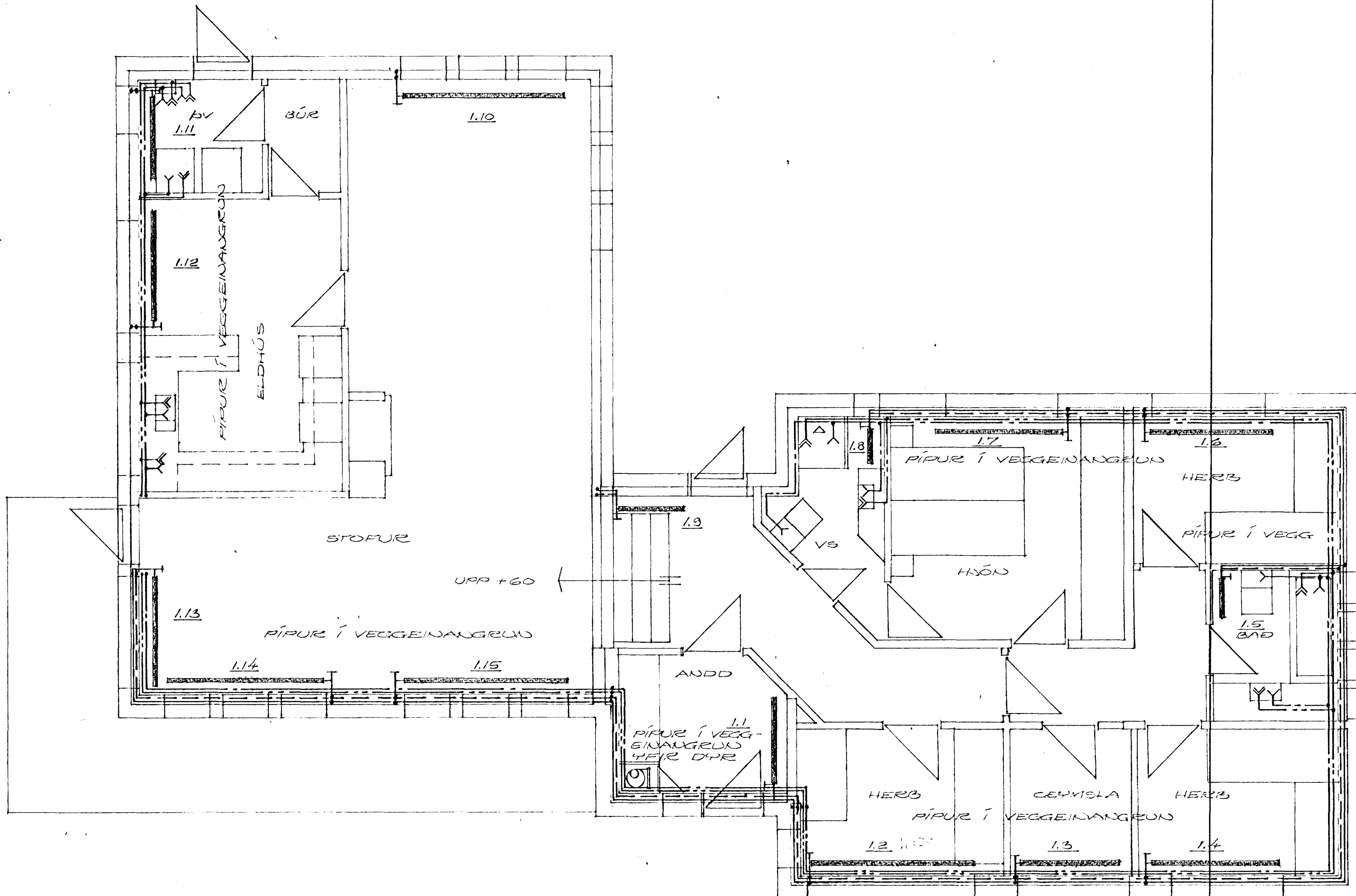
GRUNNMYND EFRÍ HÆÐAR, M=1:50
