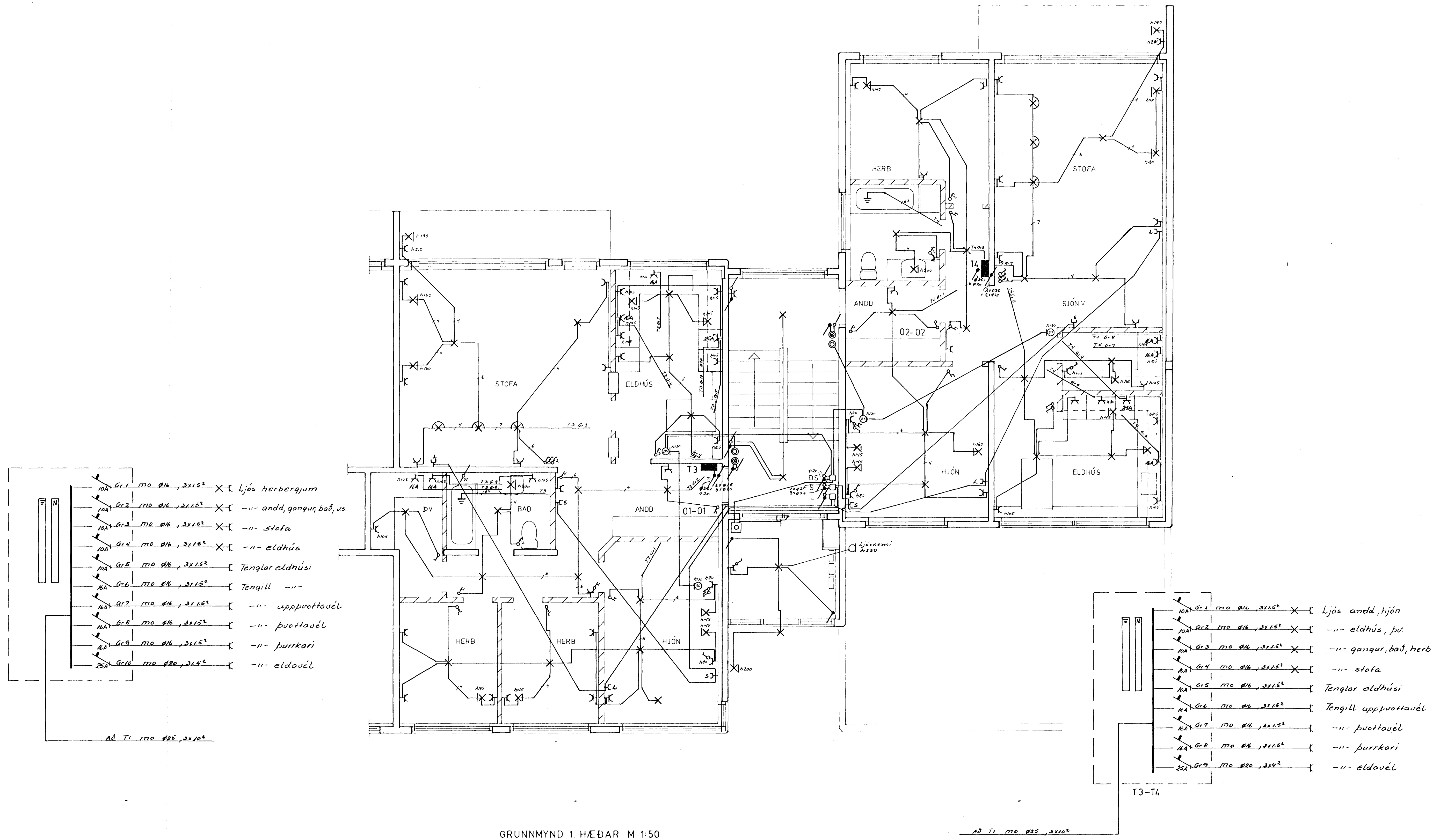
GRUNNMYND 1. HÆÐAR M 1:50
