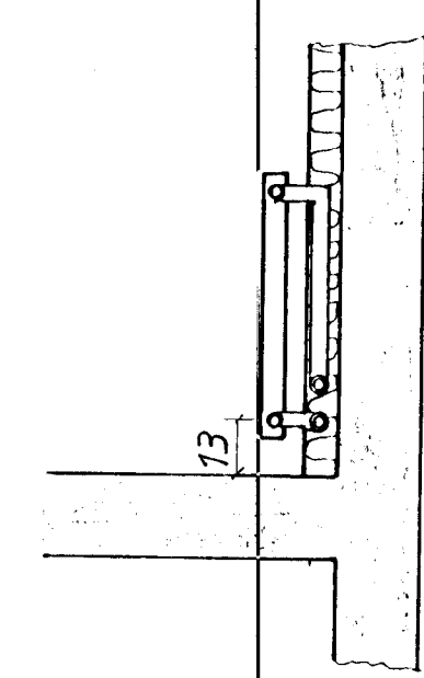
Snið C-C 1:20
