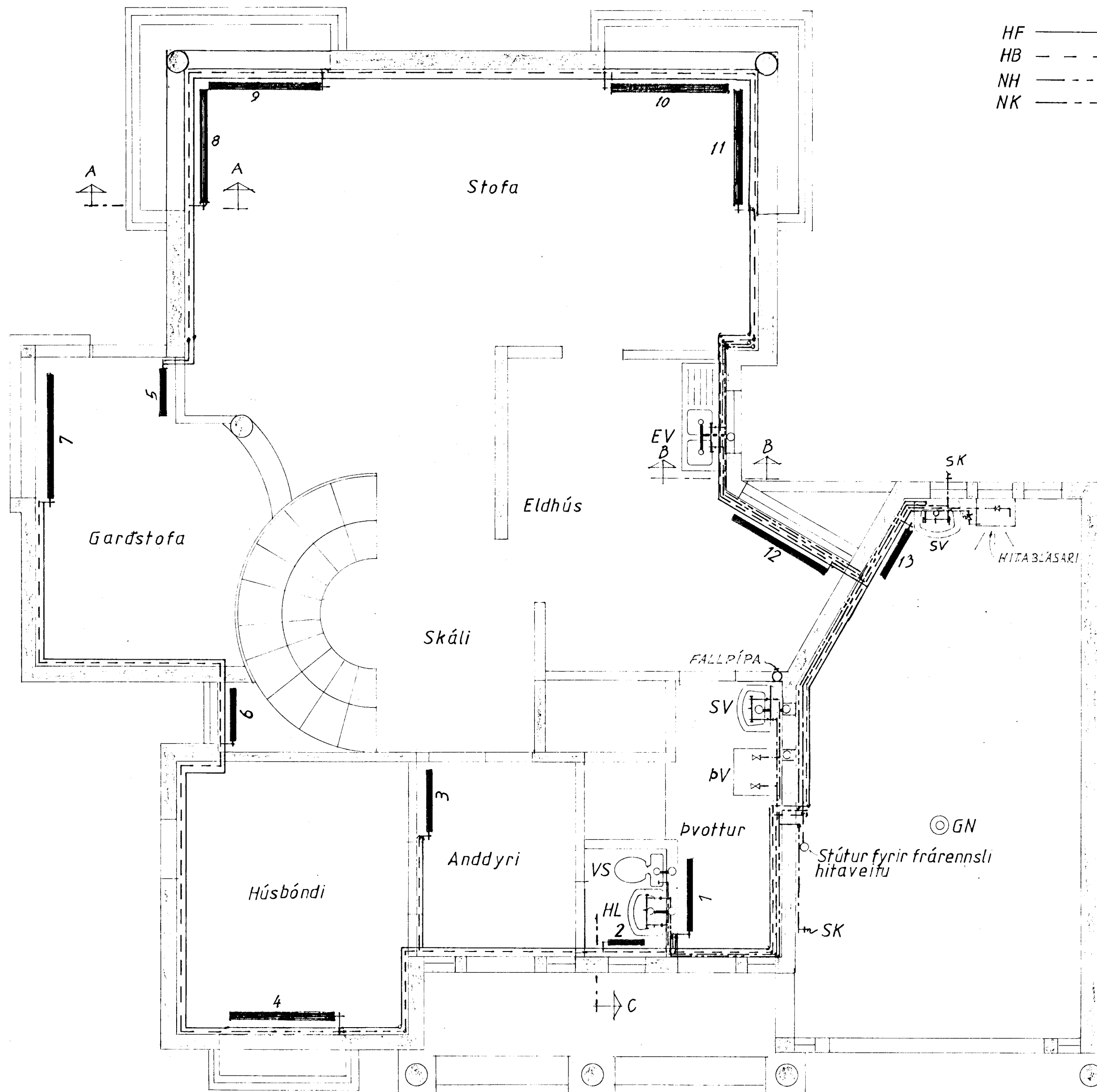
1. hæð - grunnmynd
