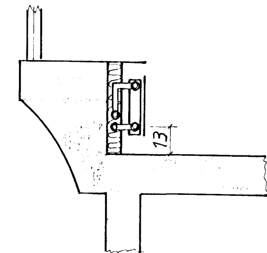
Snið A-A 1:20
