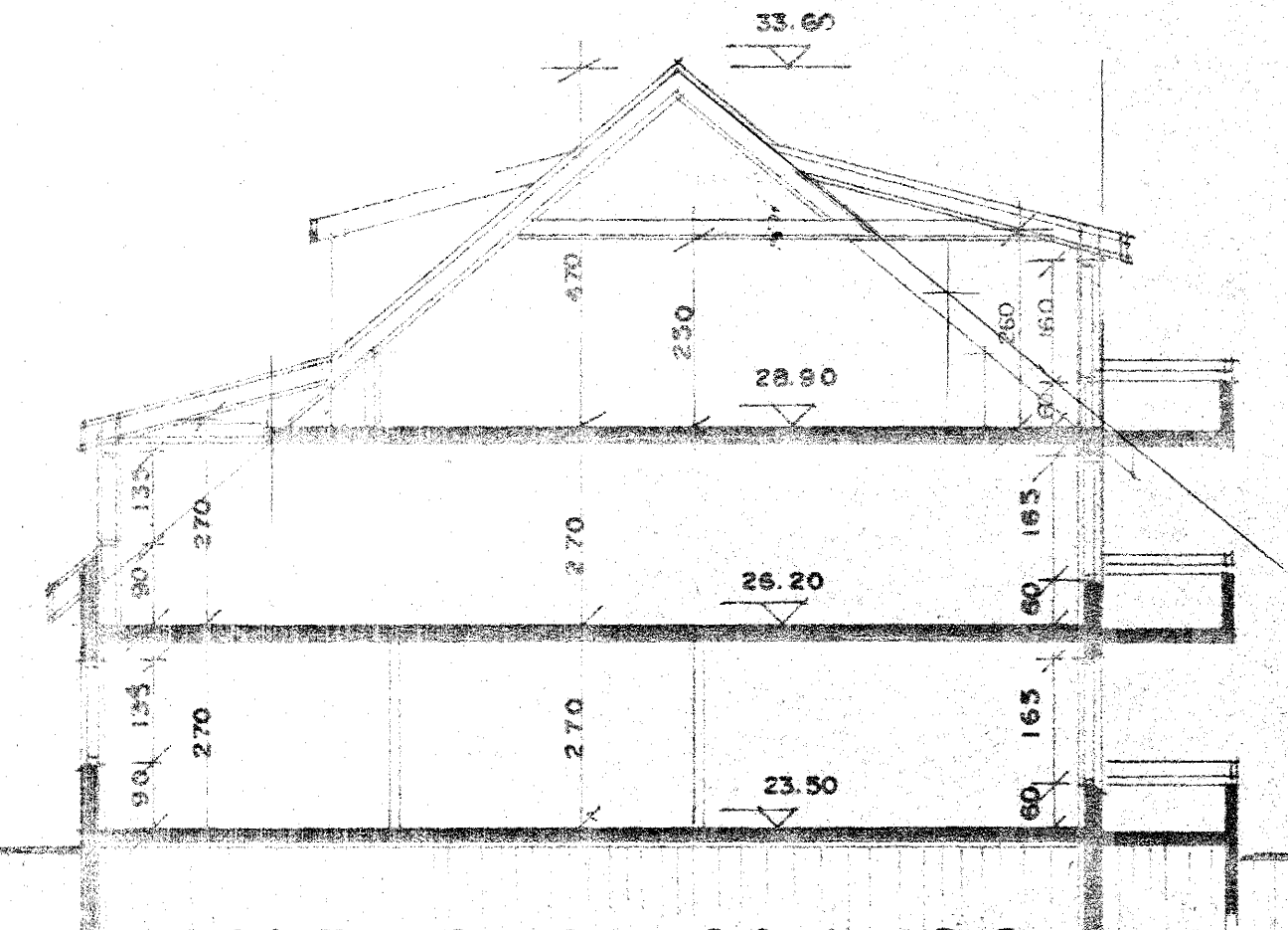
SNID A-A M. 1:100
