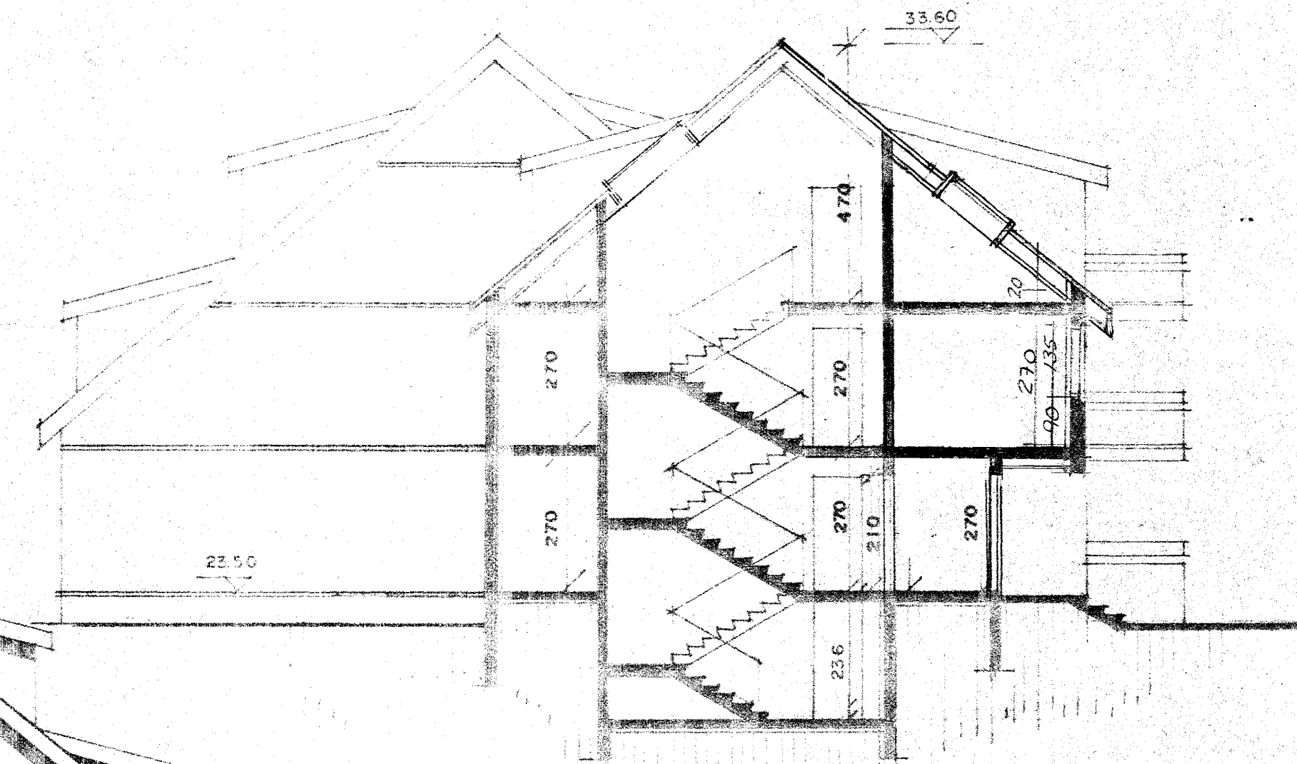
SNID B-B M. 1:100
