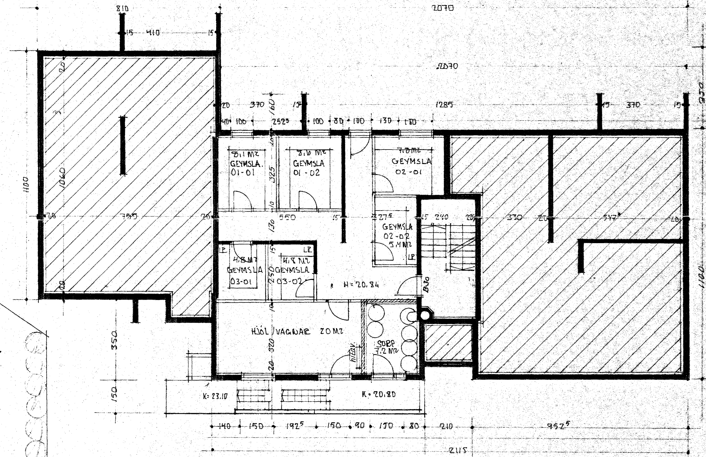
KJALLARI M. 1:100.
