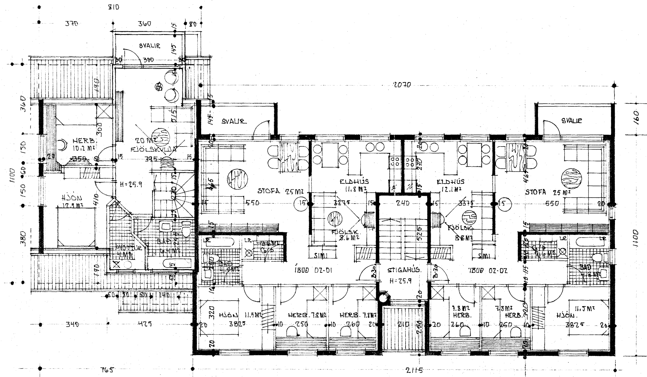
2. HÆÐ. M. 1:100
