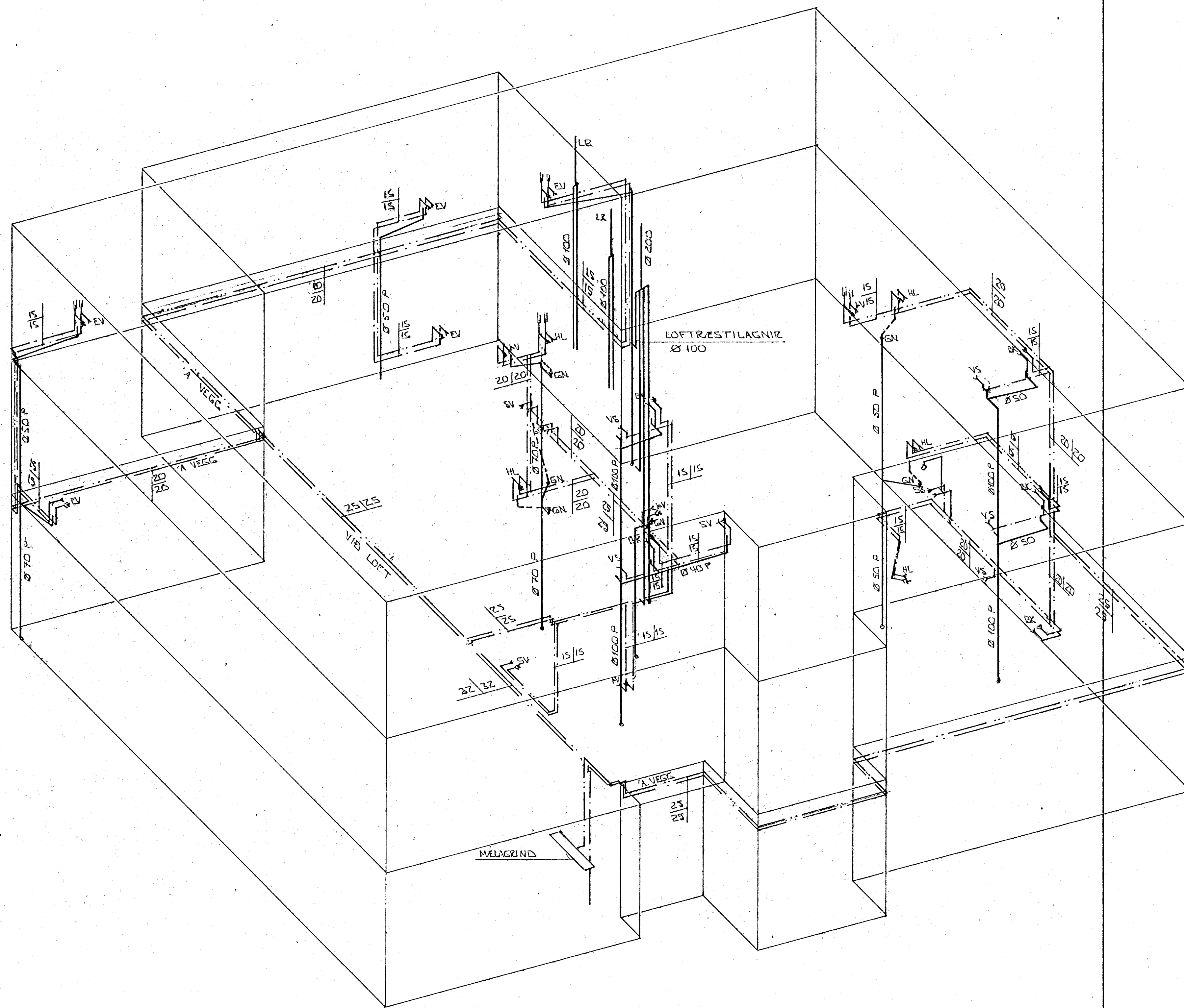
RÚMMYND 1:50
