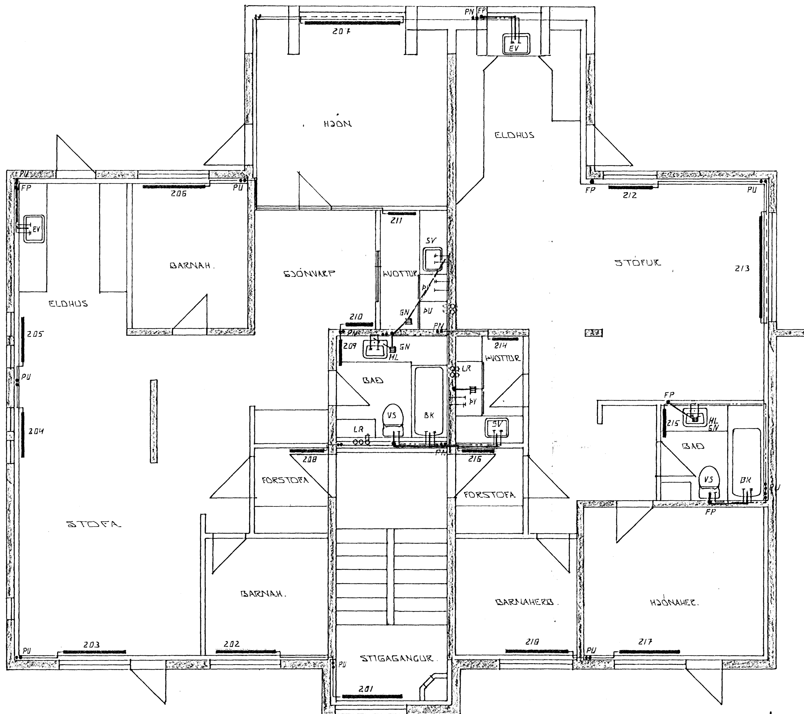
GRUNNMÝND 2. HÆÐ 1:50
