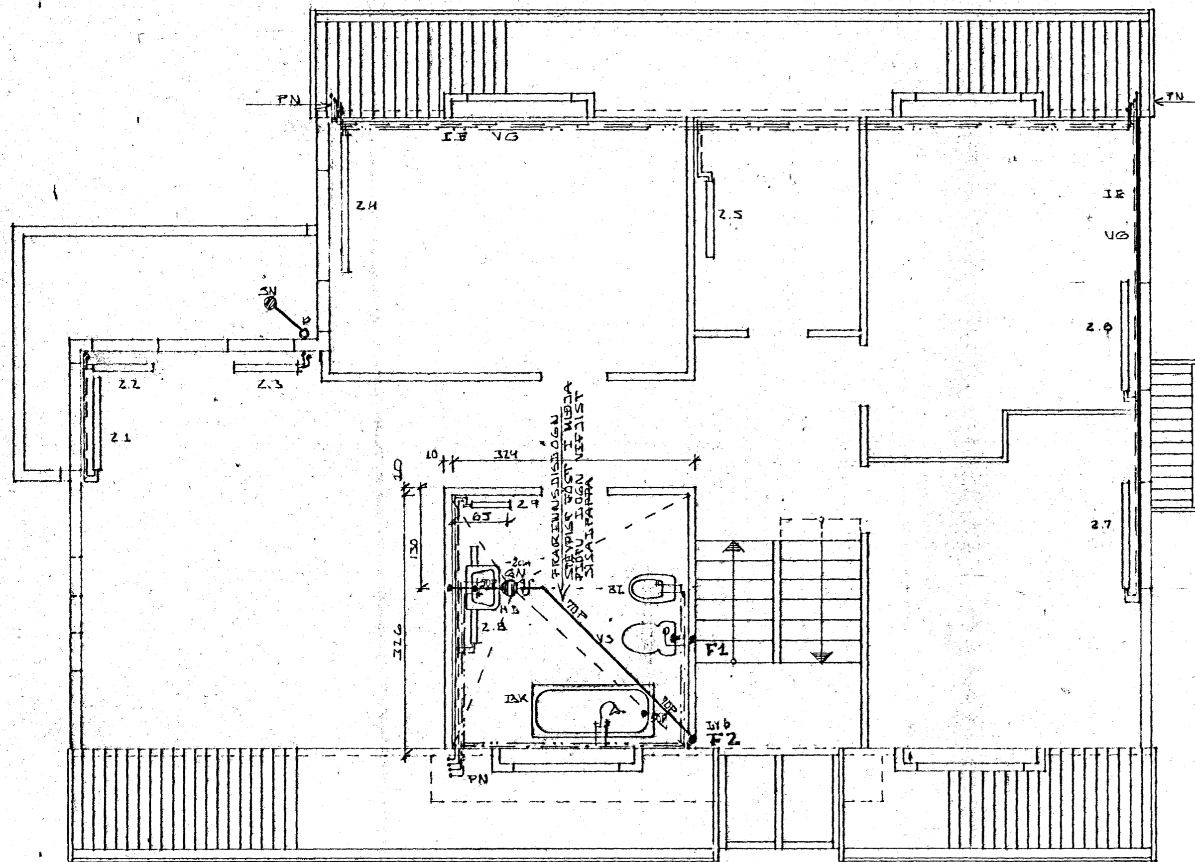
GRUNNMYND RISHÆÐAR 1:50
