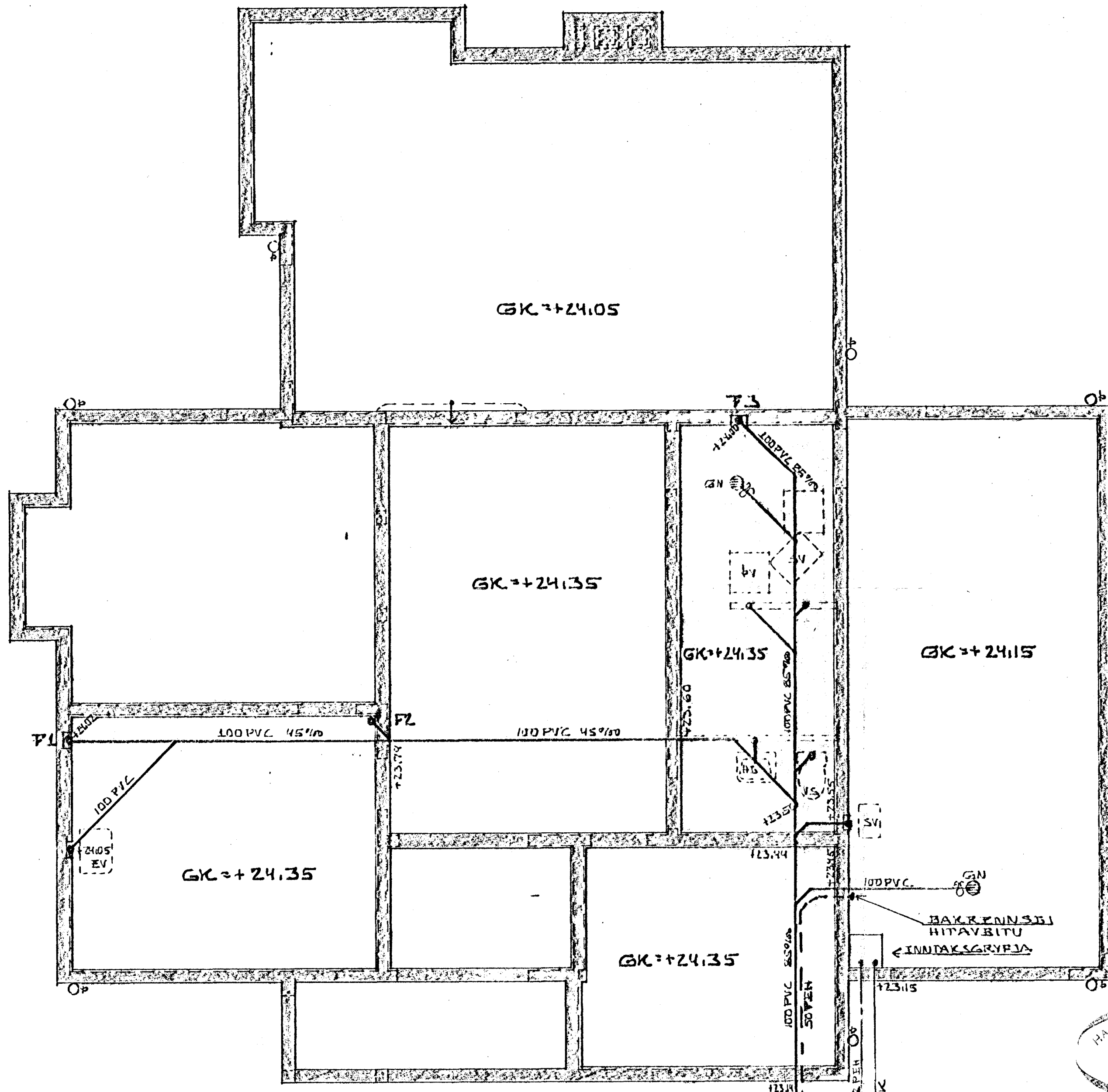
GRUNNMYND 1:50
