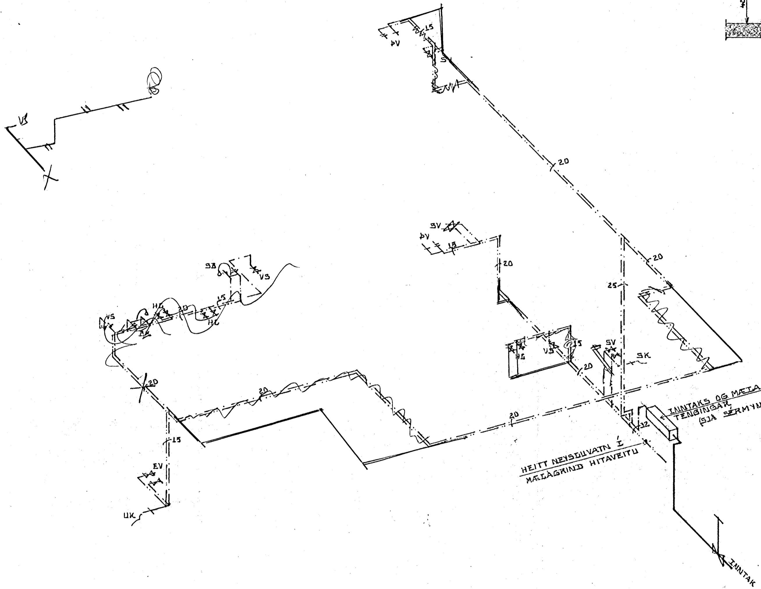
KERFISMYND VATNSLAGNA 1:50
