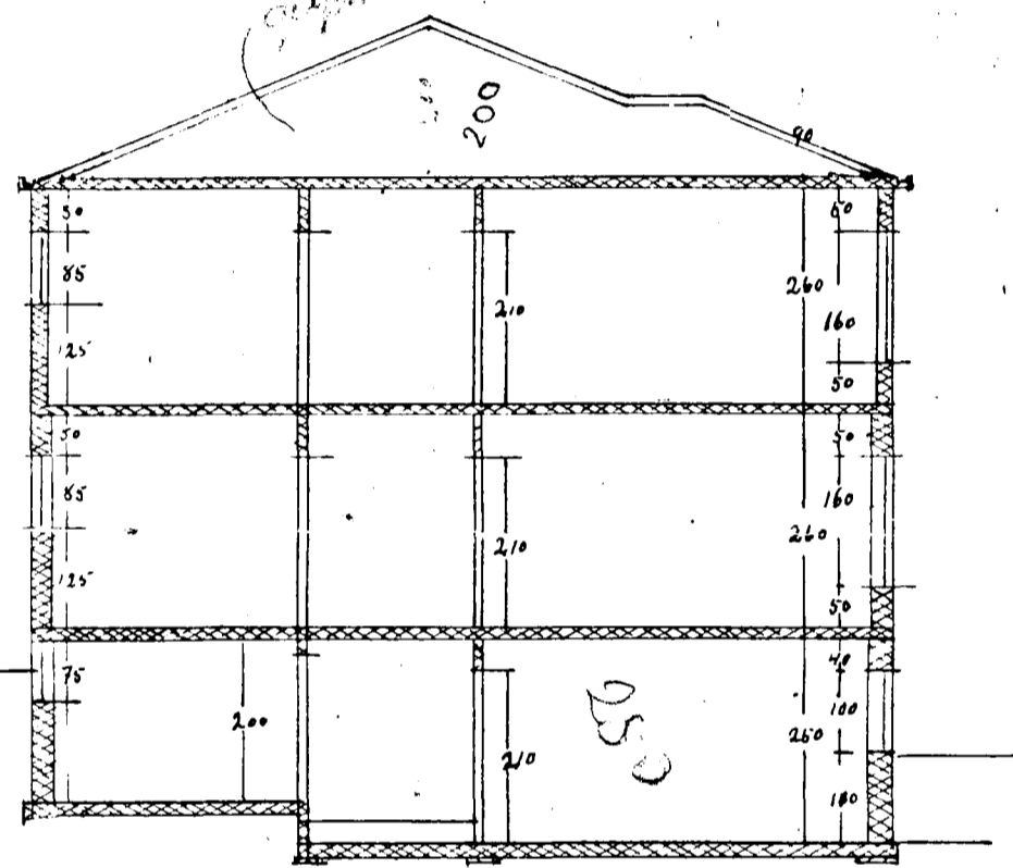
SKURÐUR A-A
