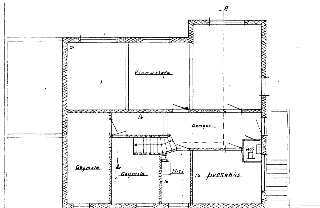
KJALLARI
