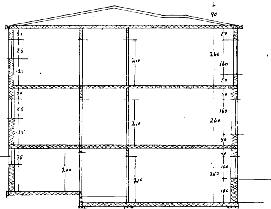
SKURÐUR A-A
