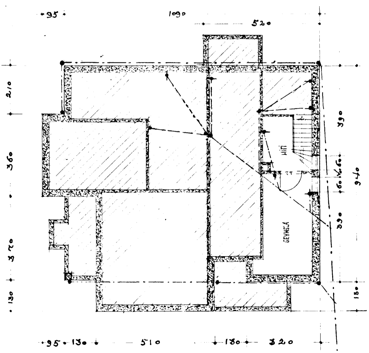
UNDIRSTÖÐUR
