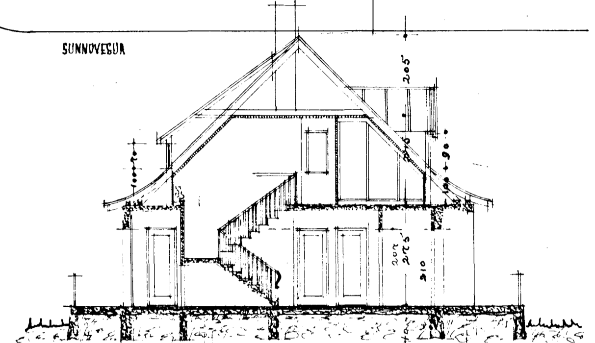
SKURÐUR
