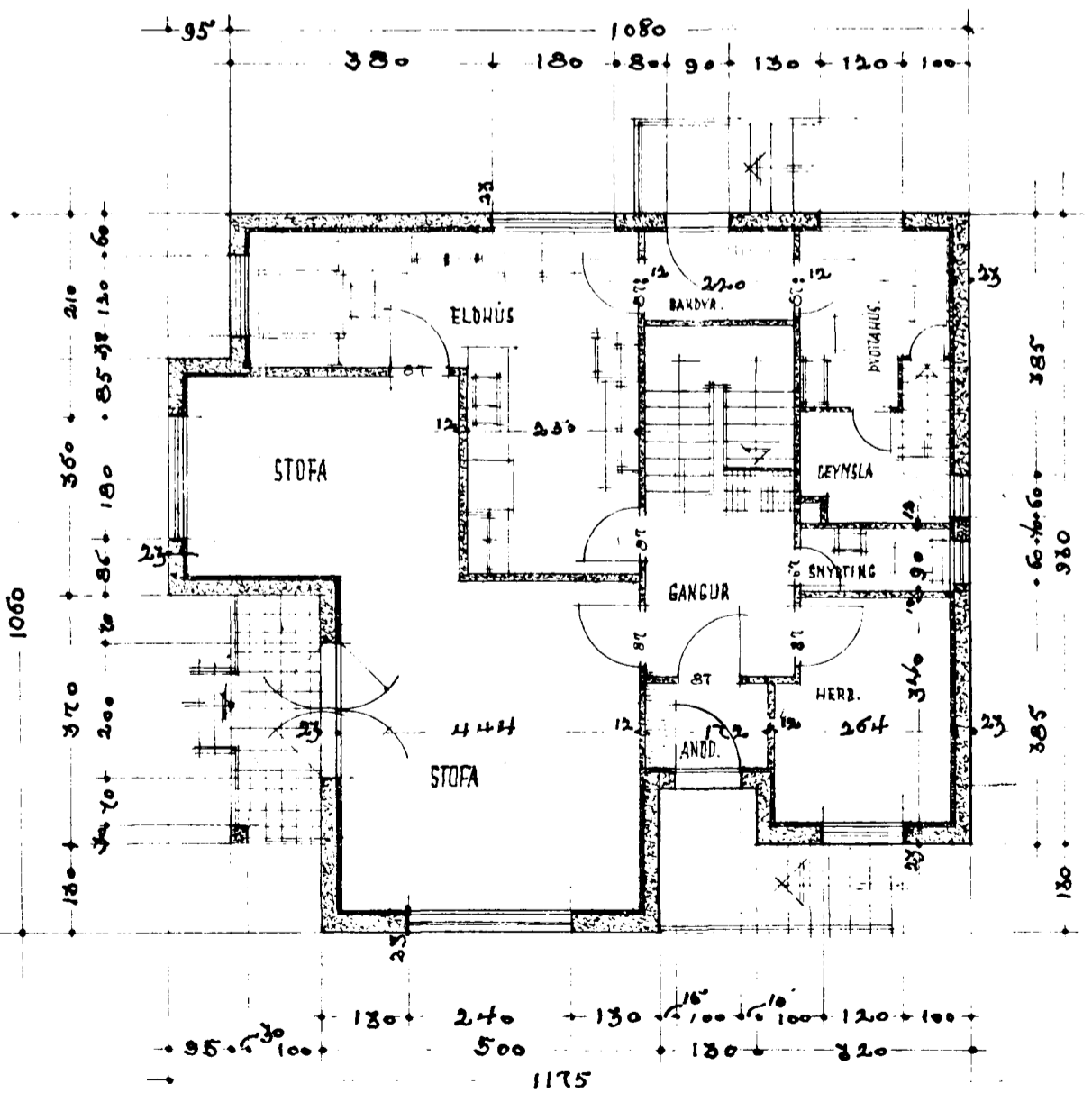
HÆÐIN
