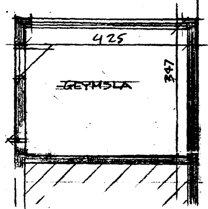
GRUNNMYND KJALLARA 1:100
