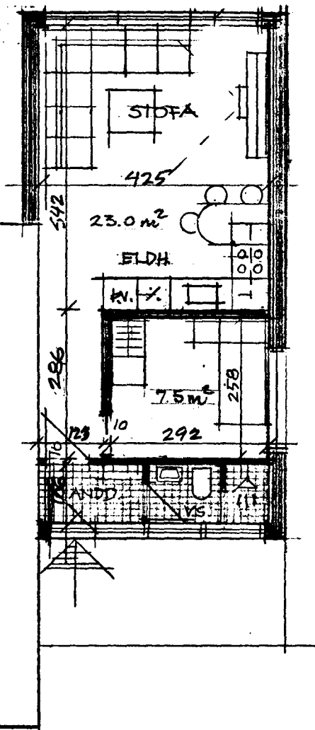
GRUNNMYND ADALHÉÐAR 1:100
