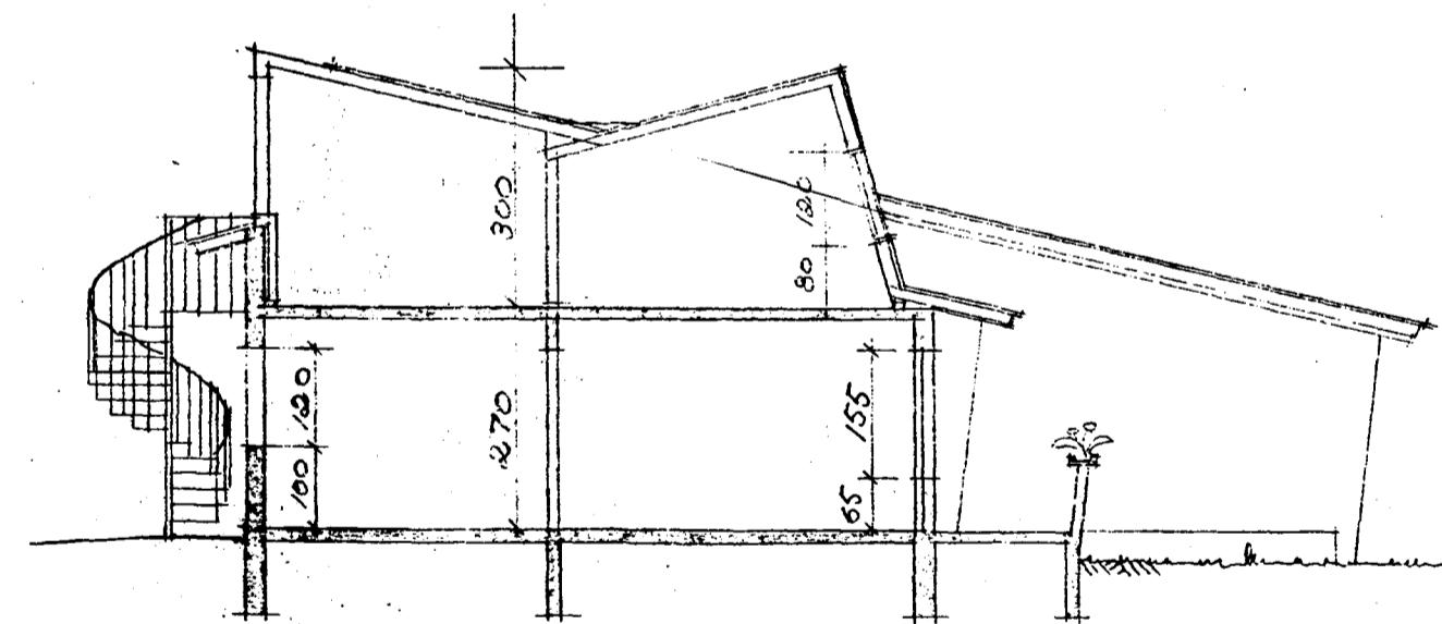
SNEIÐING
