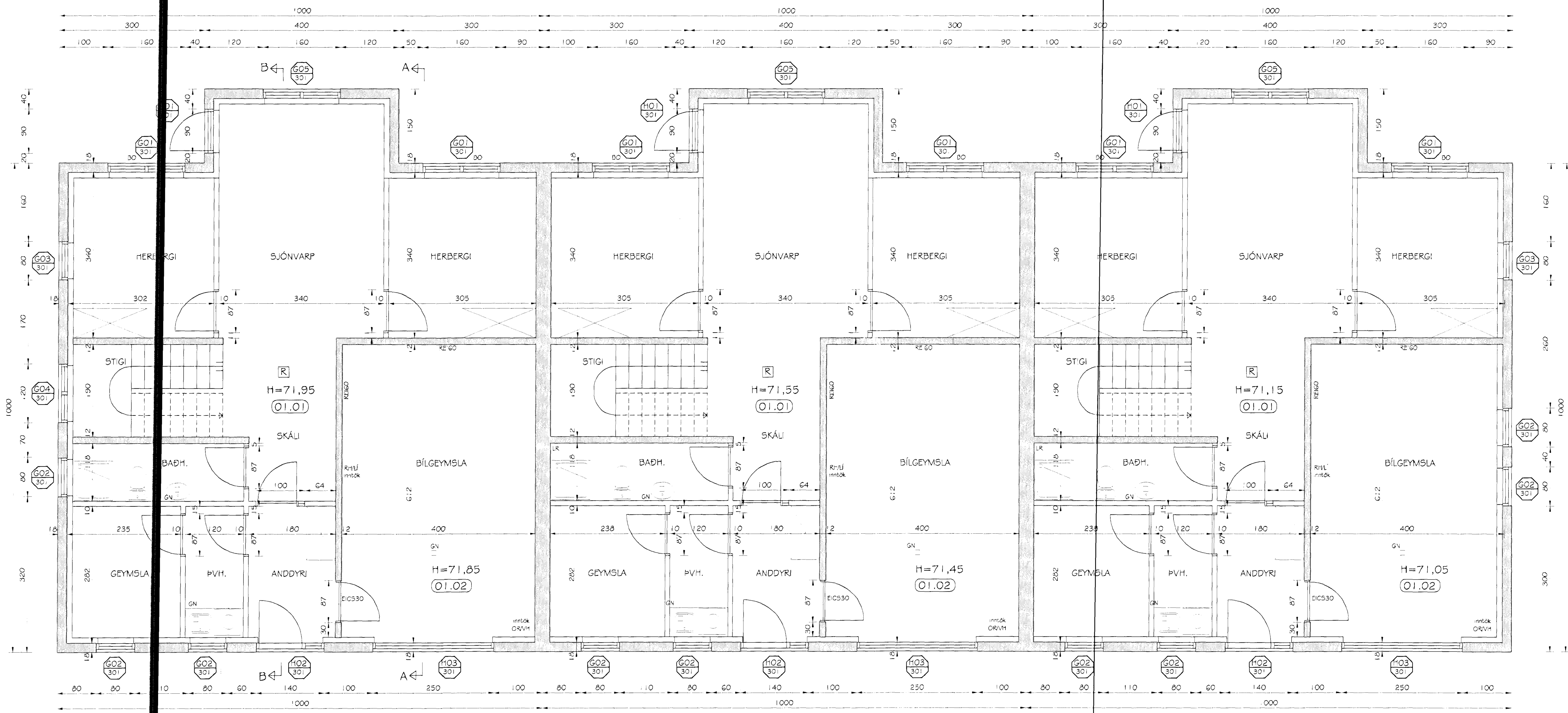
GRUNNMÝND NEDRI HÆÐAR MKV. 1:50
