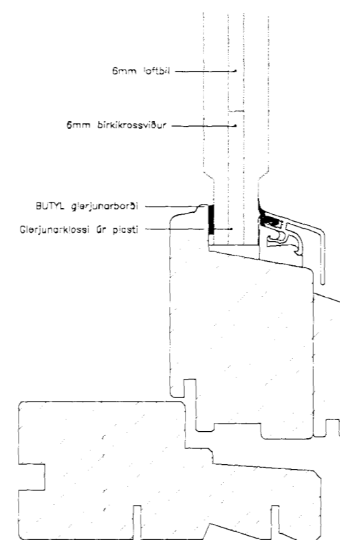
UNDIRSTYKKI Í SVALAHURÐ
