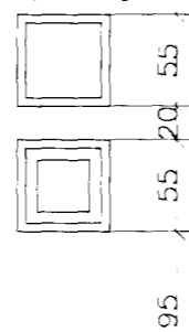
gluggi g-3 10 stk.+ 14 stk.opnanlegir
