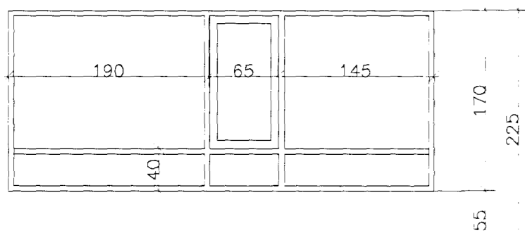
gluggi g-1 1 stk.
