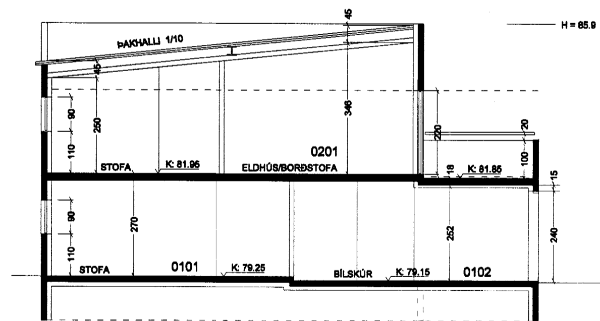
SNEIÐ C - C
