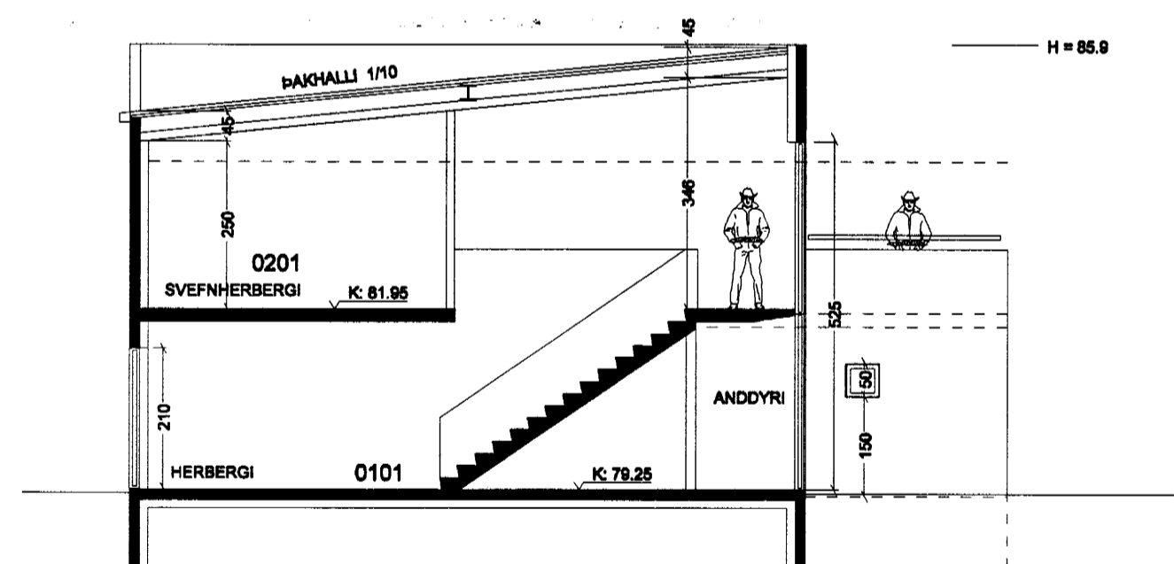
SNEIÐ B - B
