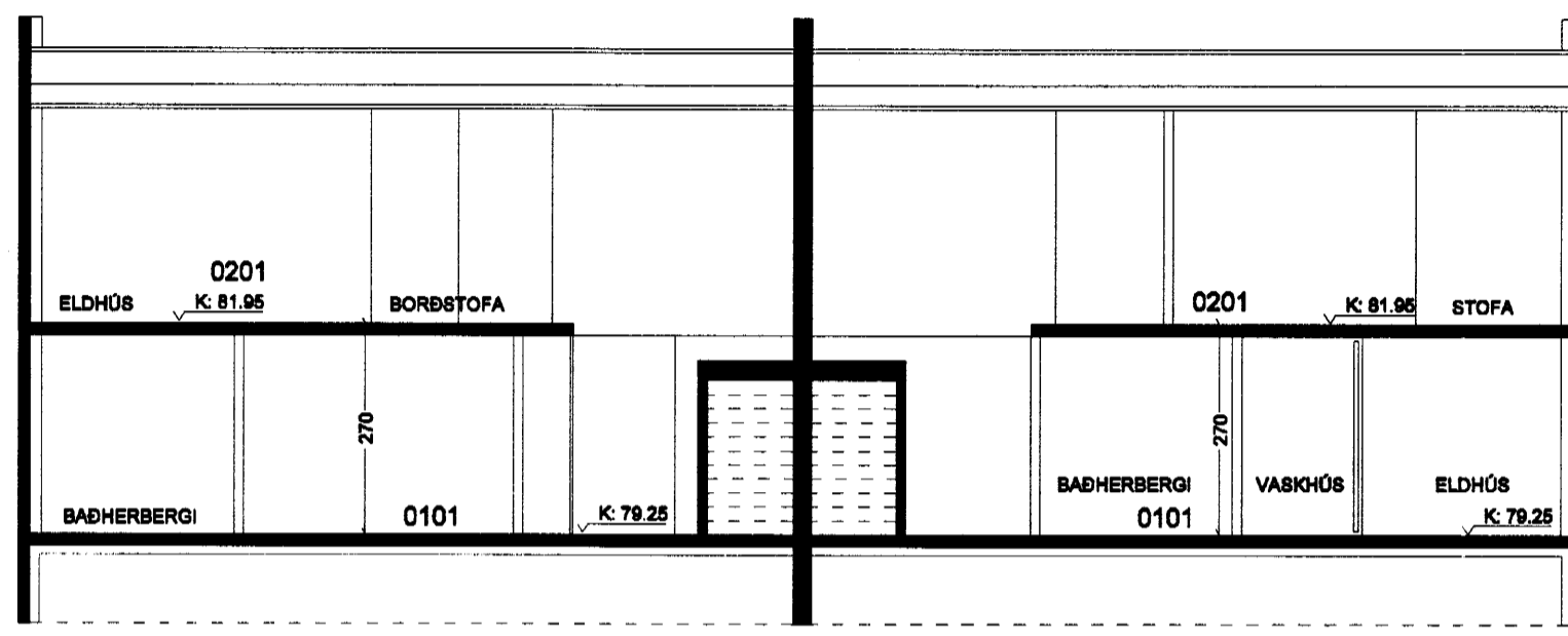
SNEIÐ A - A
