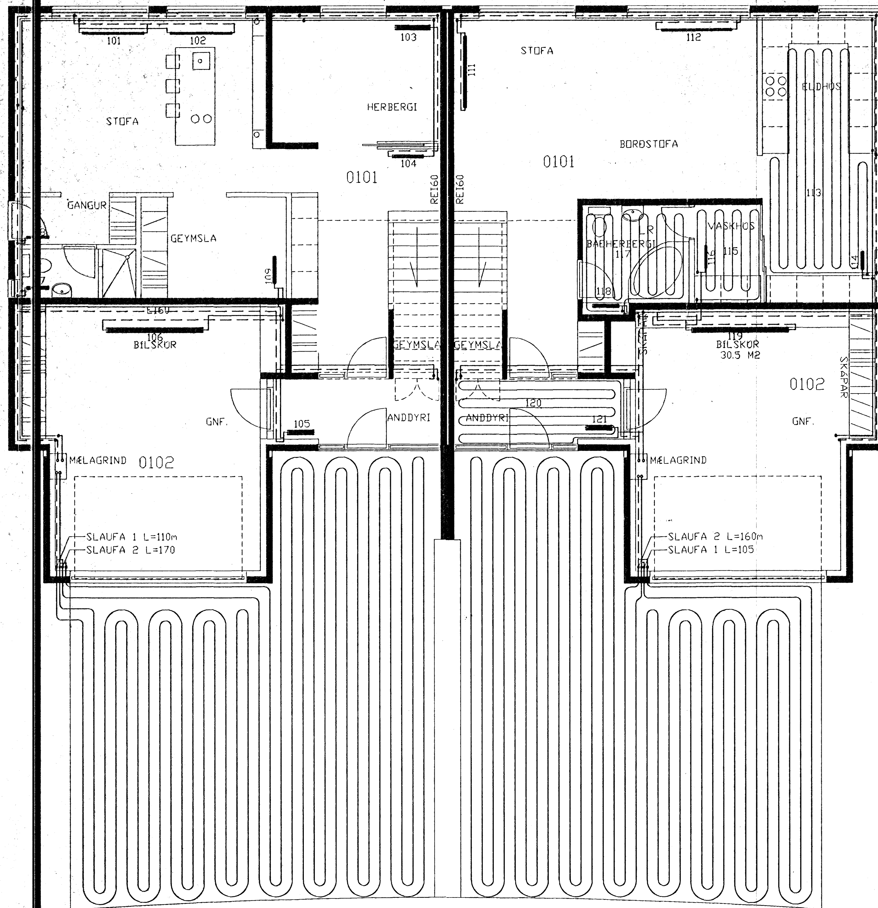
GRUNNMYND 1. HÆÐ HITAKERFI
