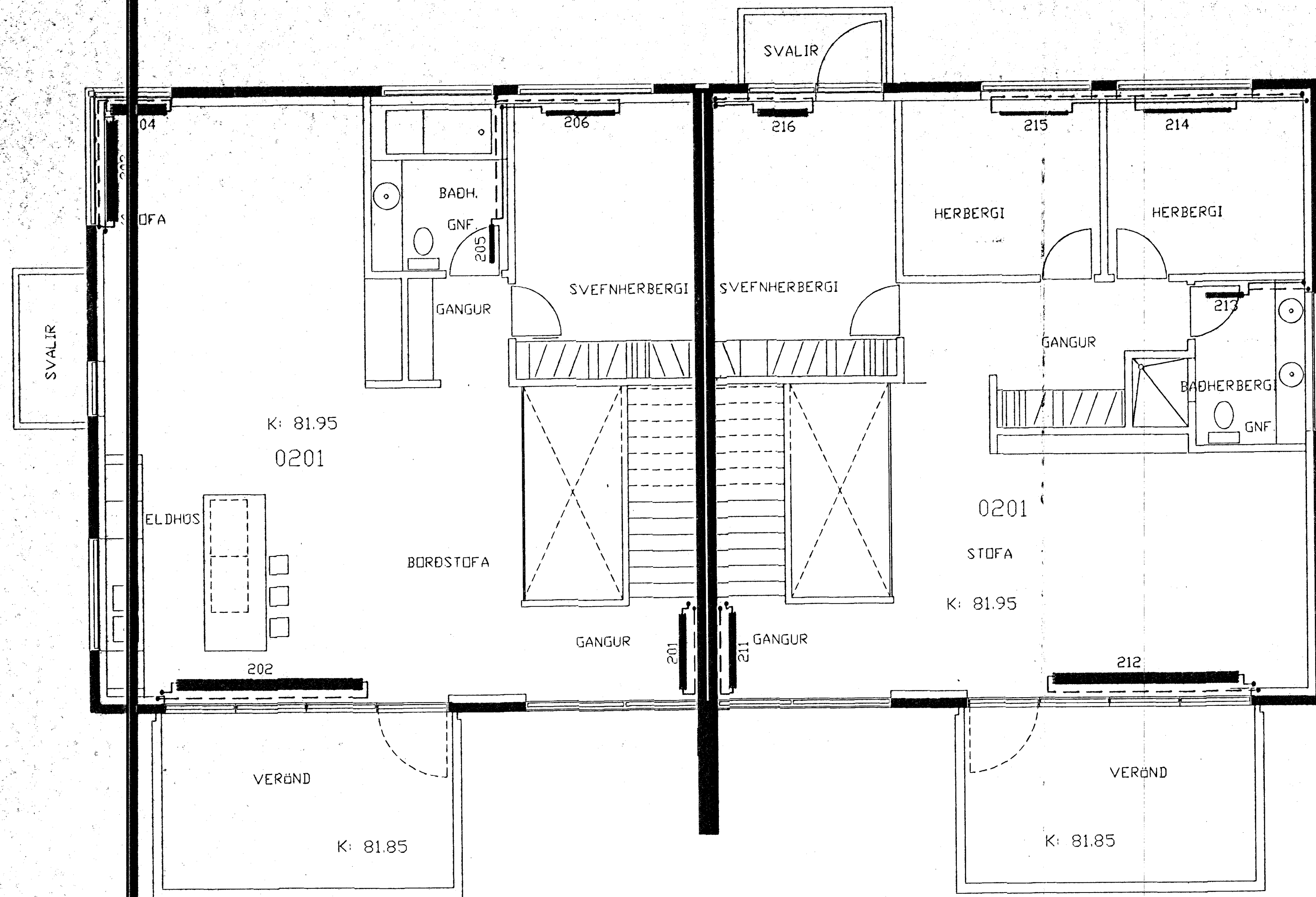
GRUNNMYND 2. HÆÐ HITALAGNIR
