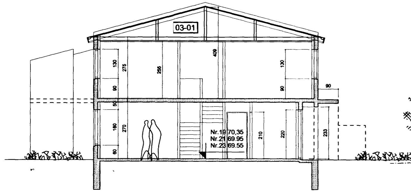
SNID B - B 1 : 100
