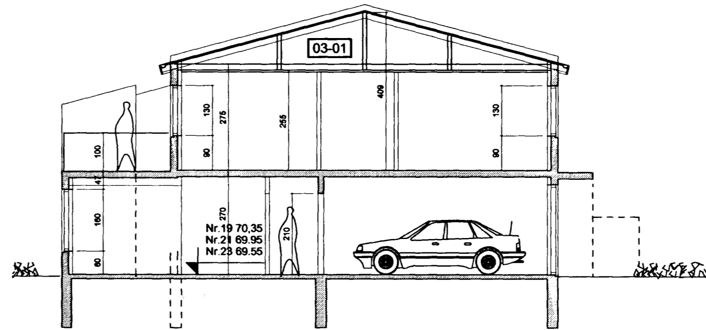
SNID A - A 1 : 100
