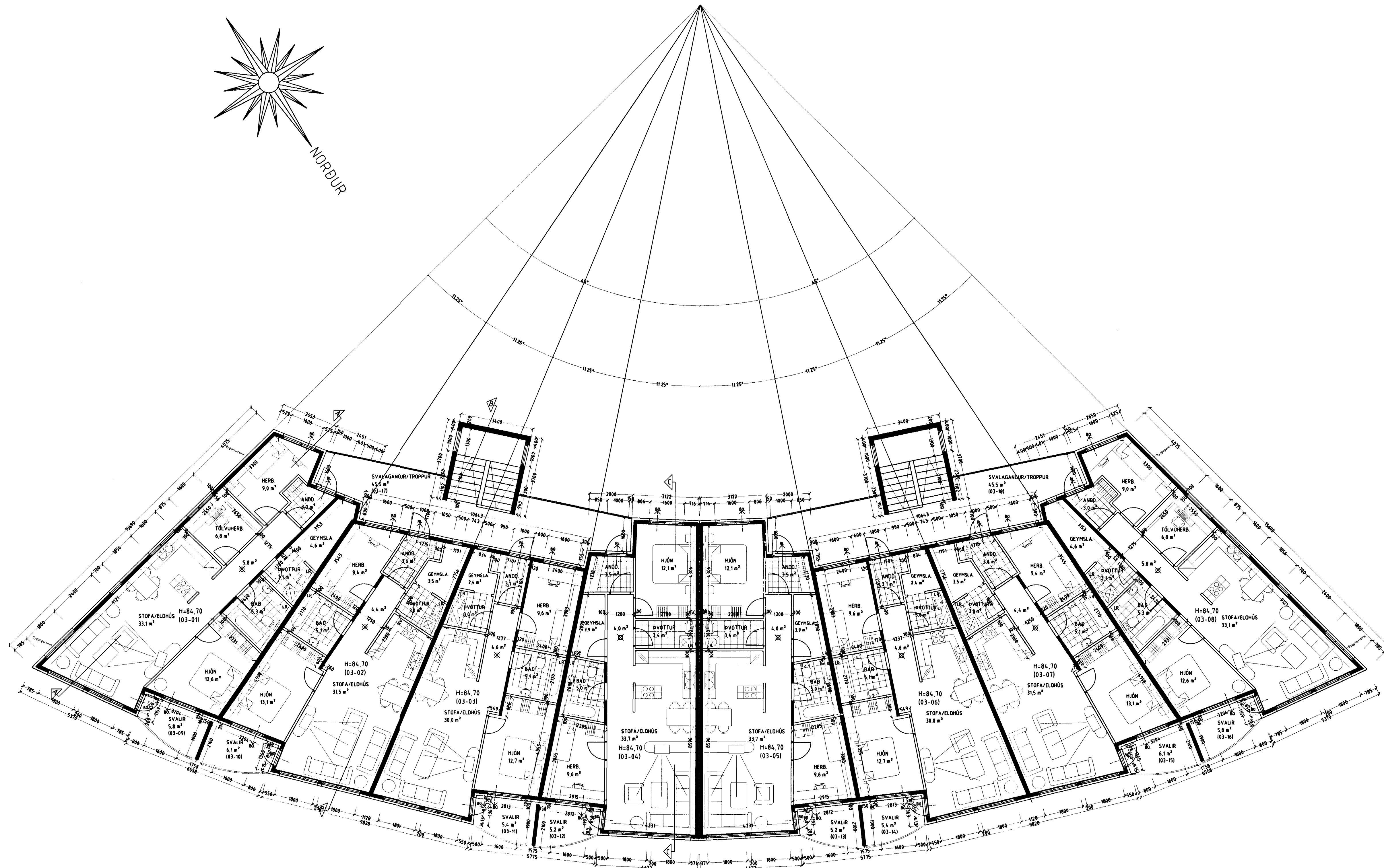
GRUNNMYND 3 HÆÐ. MKV. 1:100.
