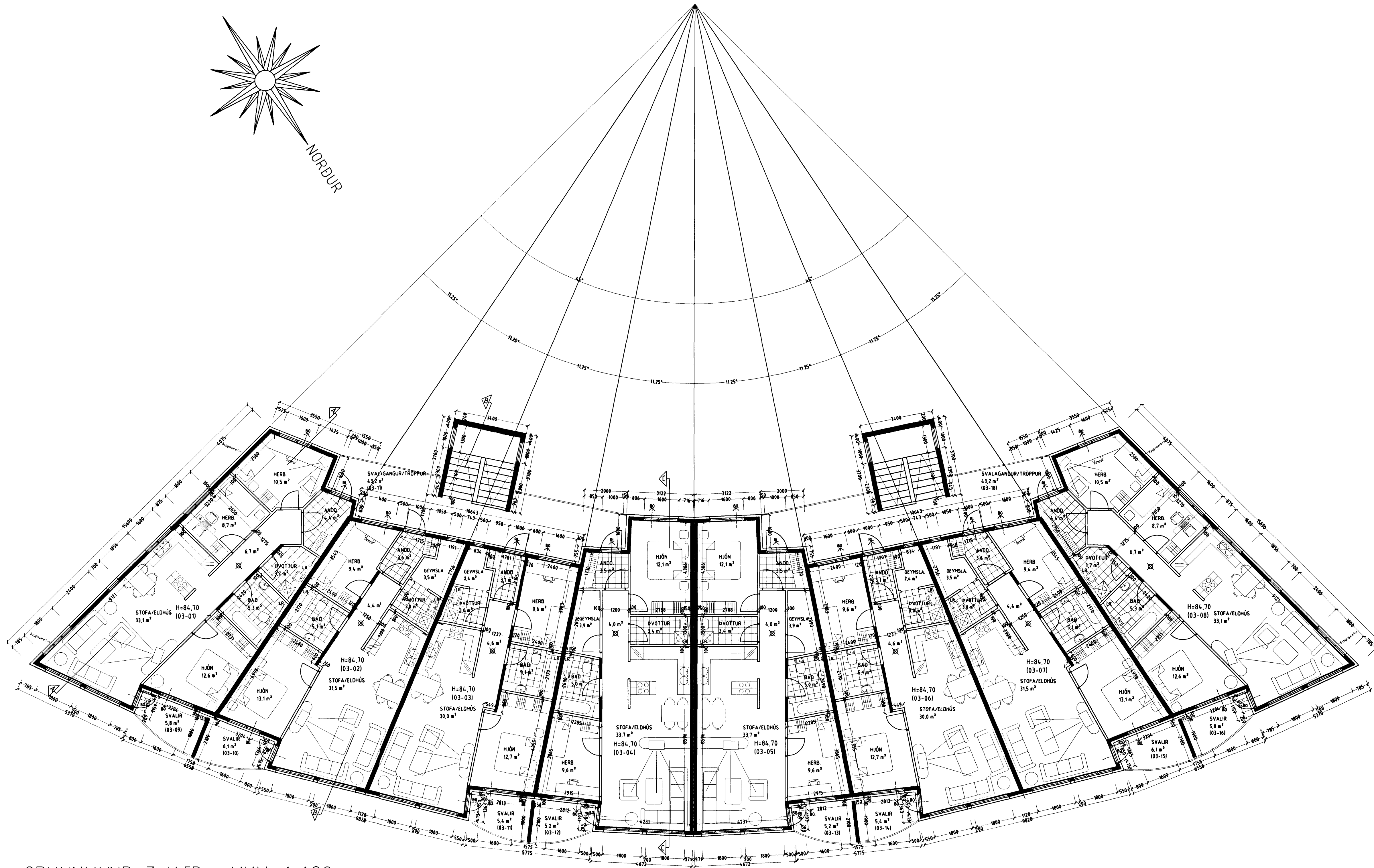
GRUNNMYND 3 HÆÐ. MKV. 1:100.
